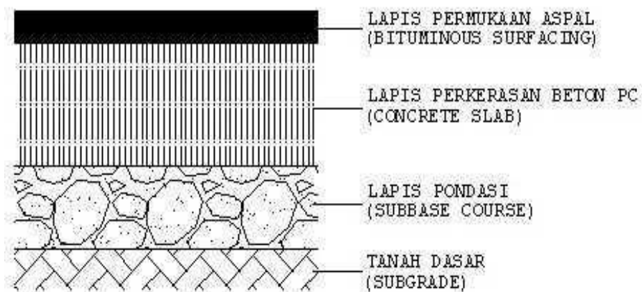
Gambar 2.3. Lapis perkerasan komposit ( Composite Pavement )
