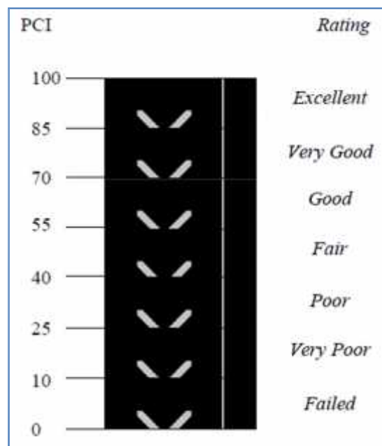
Gambar 2.5 Rating Kondisi Perkerasan Berdasarkan Nilai PCI
