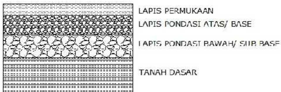
Gambar 2.4 Bagian Lapisan Konstruksi Perkerasan Jalan
