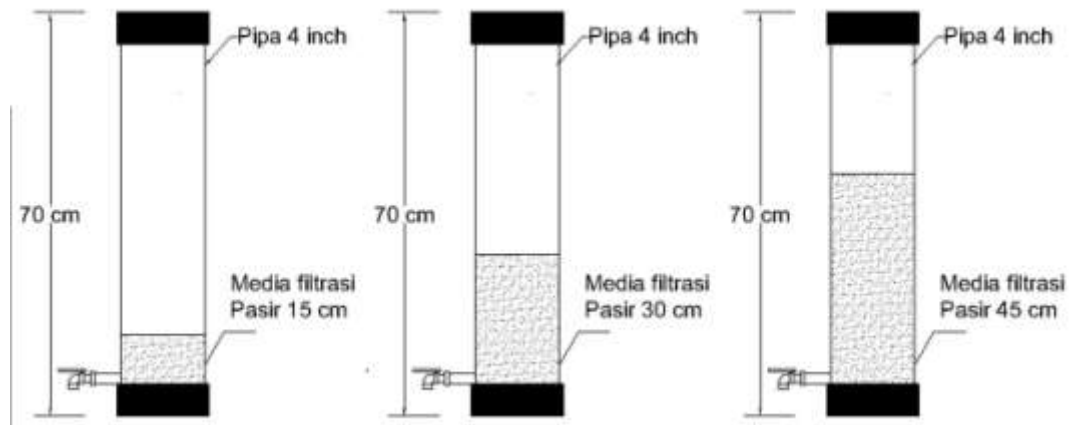
Gambar 4.3 Alat uji model filtrasi media filtrasi pasir
