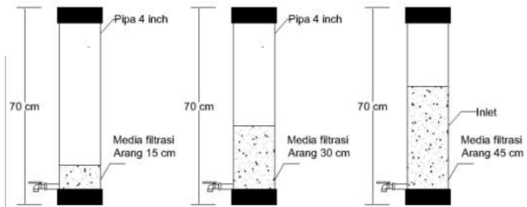
Gambar 4.5 Alat Uji Model Filtrasi Media Filtrasi Arang Batok.
