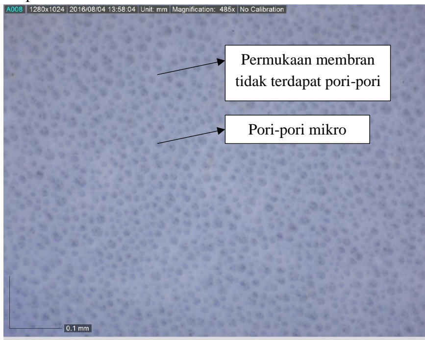
Gambar karakteristik pori-pori yang terbentuk pada membran dengan media gelatin NMP 8%
