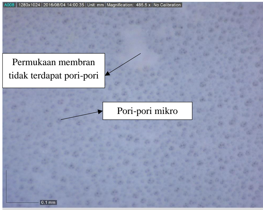
Gambar karakteristik pori-pori yang terbentuk pada membran dengan media gelatin akuades
