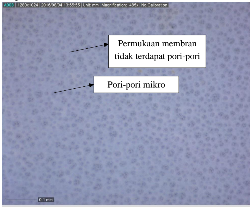
Gambar Karakteristik pori-pori yang terbentuk pada membran dengan media gelatin NMP 6%
