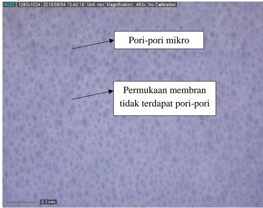
Gambar karakteristik pori-pori yang terbentuk pada membran dengan media gelatin NMP 2%
