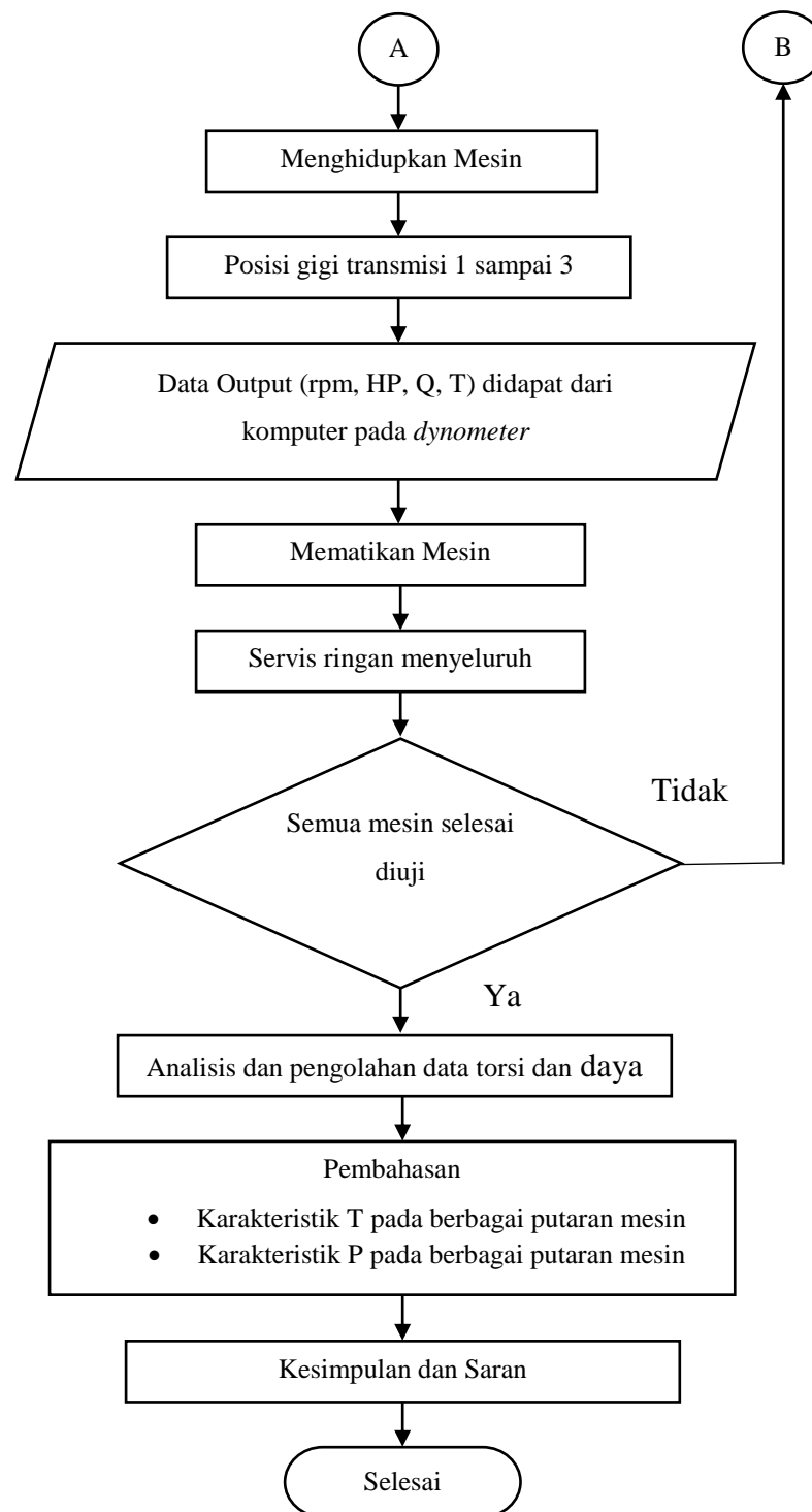
Gambar 3.19. Diagram alir pengujian Torsi dan Daya
