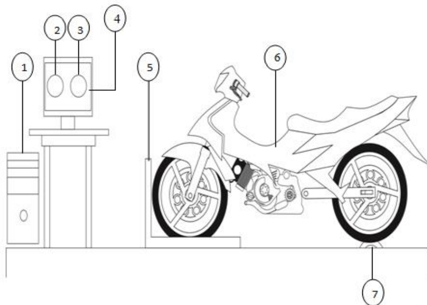
Gambar 3.17 Skema alat uji daya motor.
