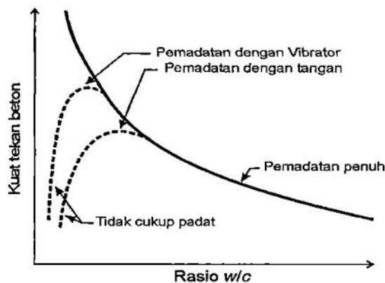
Gambar 3.1 Hubungan antara fas dan kuat tekan (Tjokrodimuljo, 2007)
