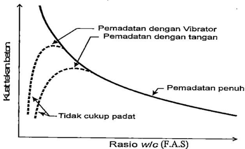
Gambar 3.3 Hubungan Antara Kuat Tekan dan Fas (w/c)
