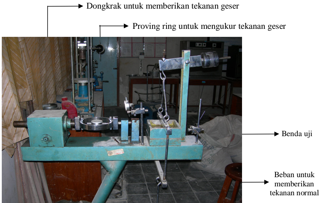
Gambar 2. Alat uji Geser Langsung.
