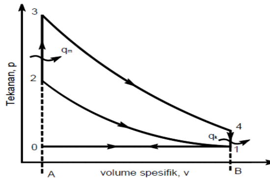
Gambar 2.2 Diagram P dan V Siklus Volume Konstan (Kristanto, 2015)
