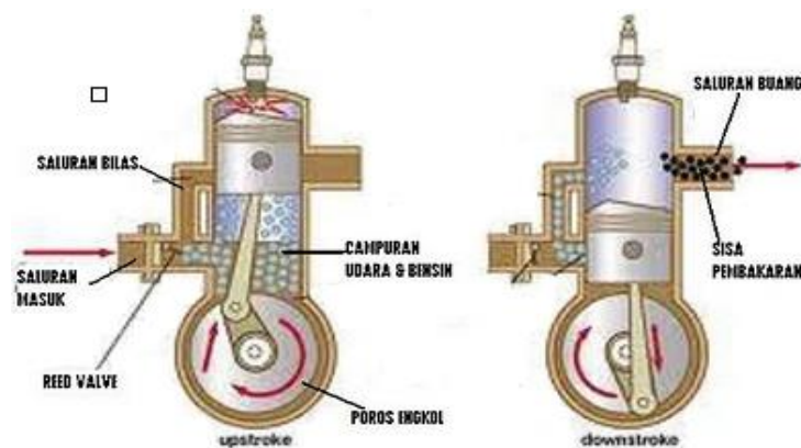
Gambar 2.4 Skema Gerakan Torak 2-Langkah (wahyu., 2013)
