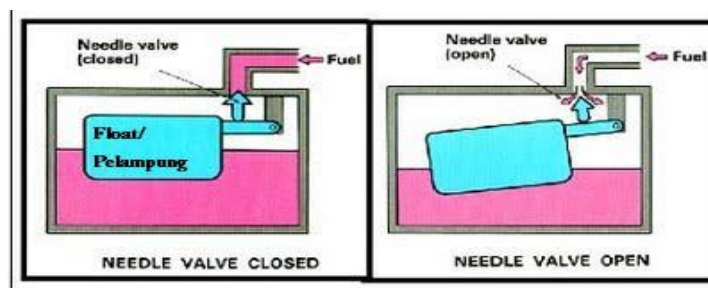
Gambar 2.18 Cara kerja pelampung dan jarum karburator (Sumito, 2013)
