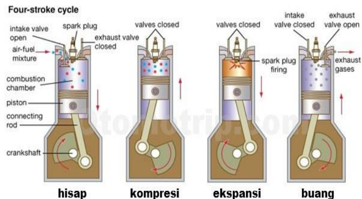
Gambar 2.3 Skema Gerakan Torak 4-Langkah (wahyu., 2013)
