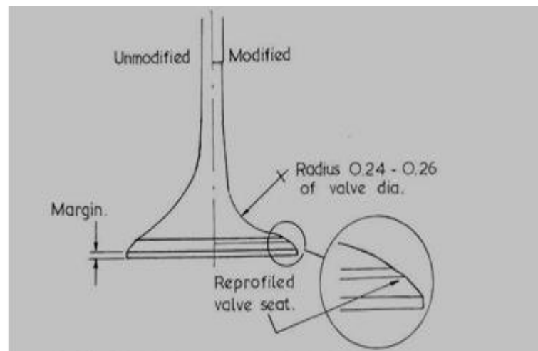
Gambar 3.9. penyudutan klep
