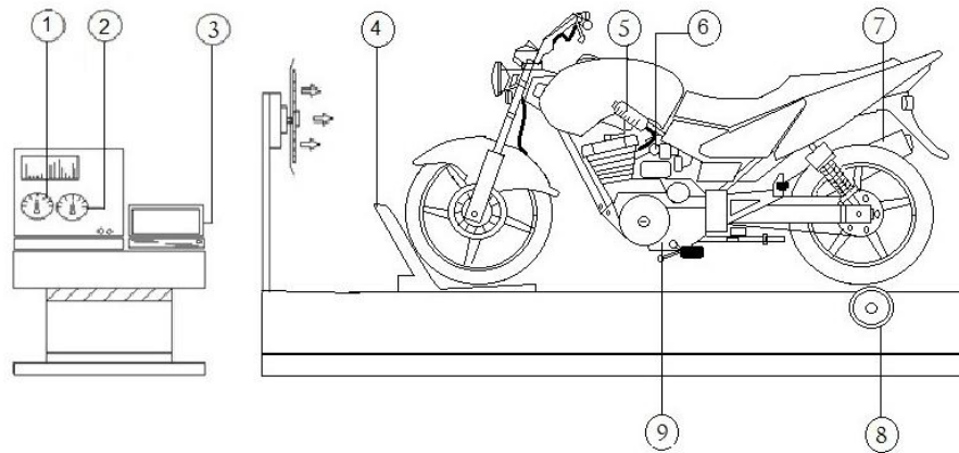
Gambar 3.10. Skema alat uji daya dan torsi motor ( Dynotest ).
