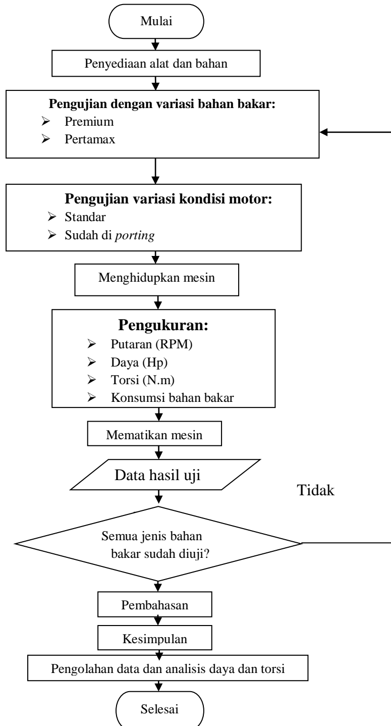
Gambar 3.6. diagram alir pengujian daya dan torsi
