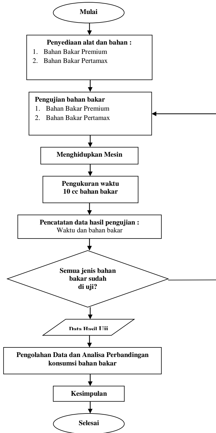
Gambar 3.7. diagram alir pengujian konsumsi bahan bakar
