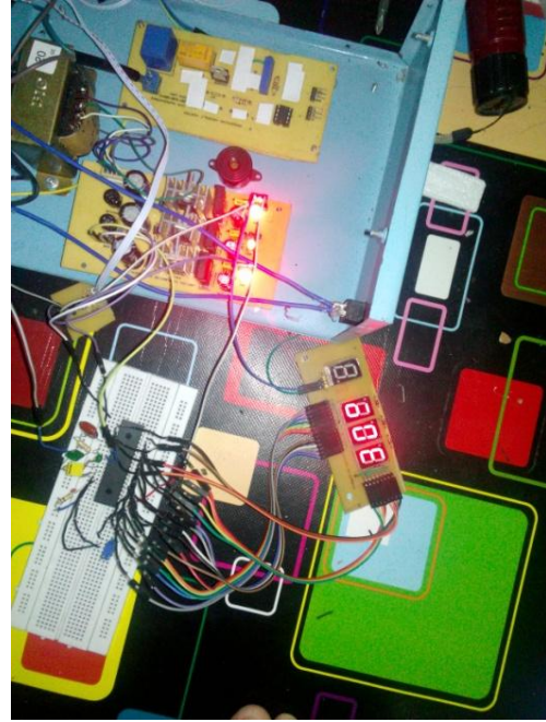
Percobaan ADC Pada Project Board
