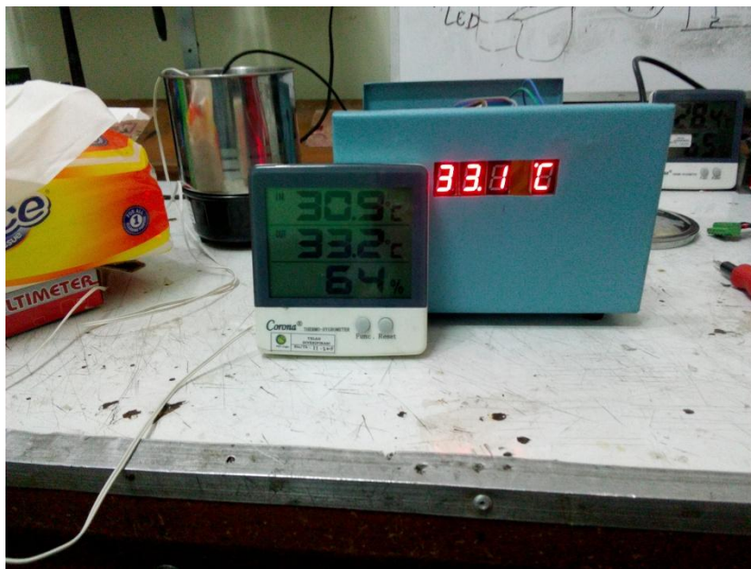
Pengkomparasian Modul Dengan Termometer Terkalibrasi
