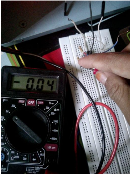
Percobaan Comparator Pada Project Board
