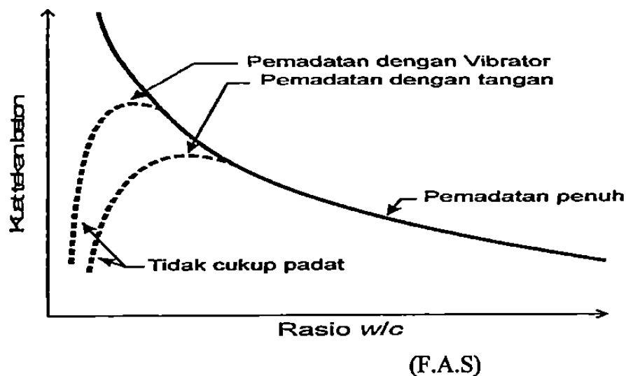
Gambar 3.2 Hubungan Antara Kuat Tekan dan Fas ( w/c ) (Tjokrodimuljo, 2007)
