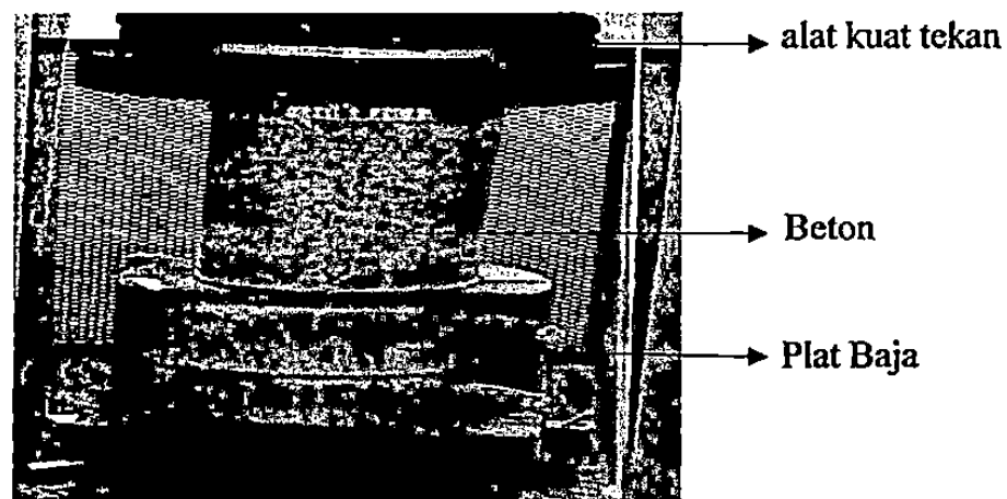
Gambar 3.1. Pengujian Kuat Tekan
