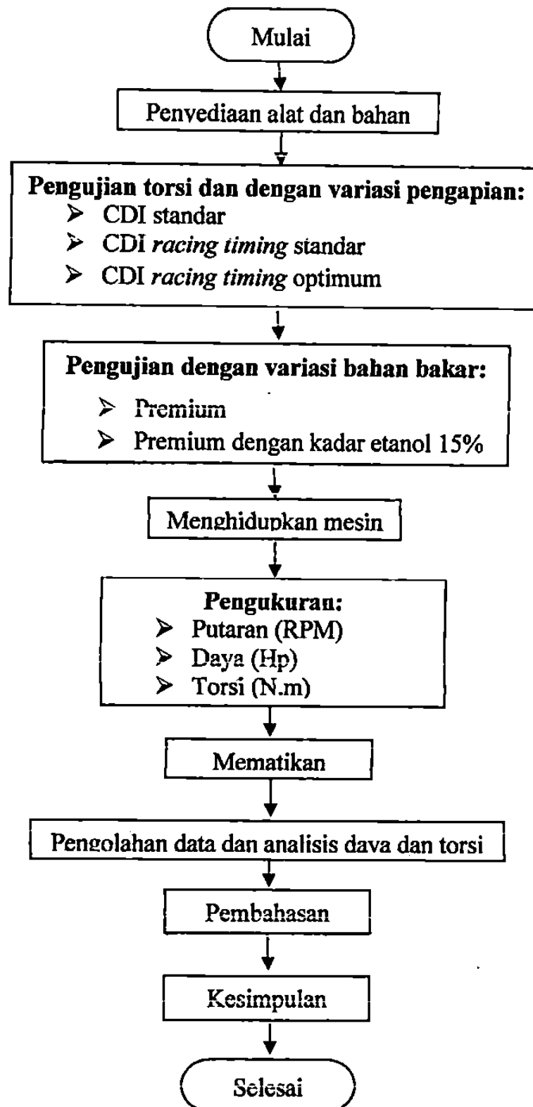
Gambar 3.6. Flow chart pengujian torsi dan daya
