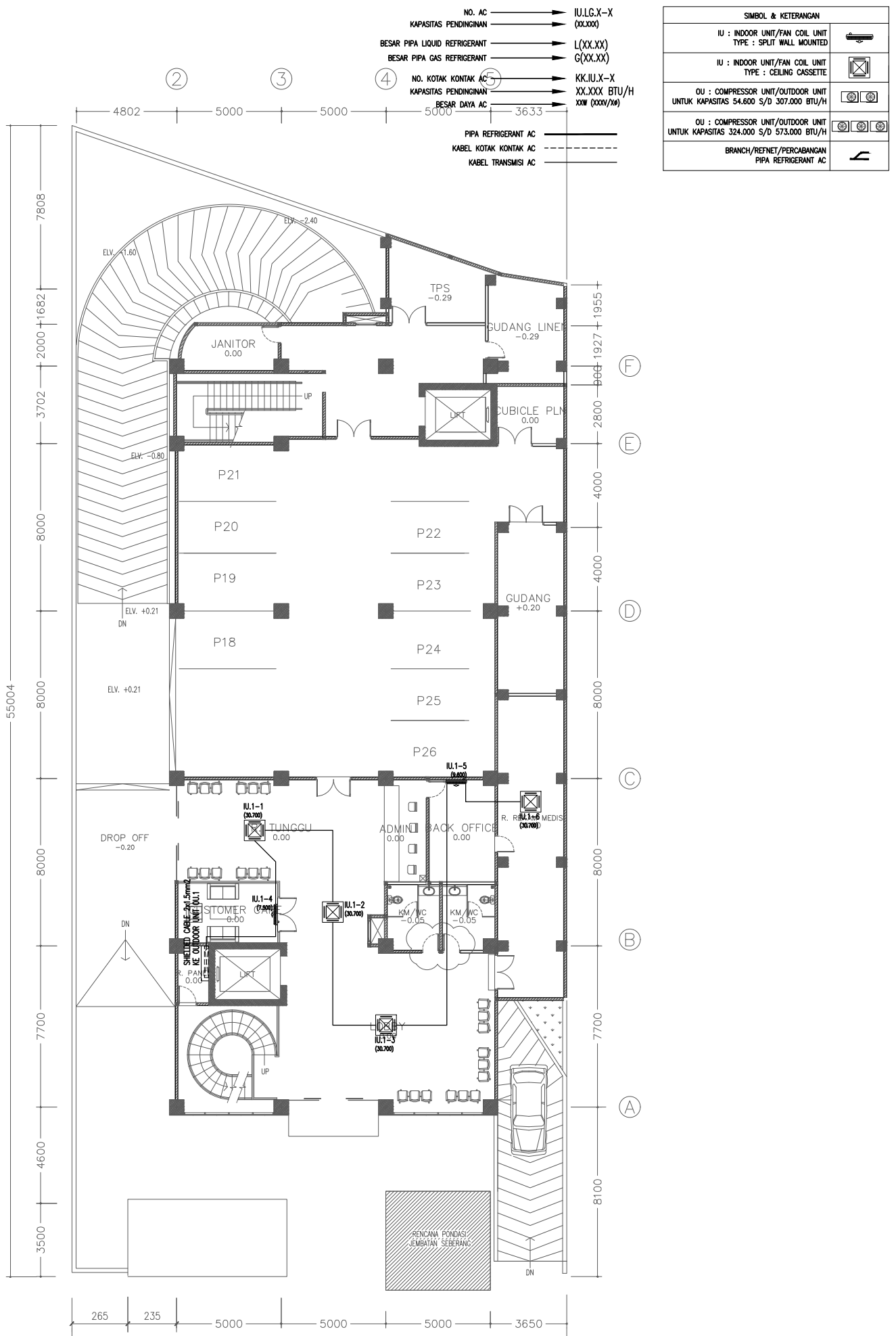
RENCANA KABEL KONTROL (TRANSMISI) AC LANTAI 1 SKALA 1:100
