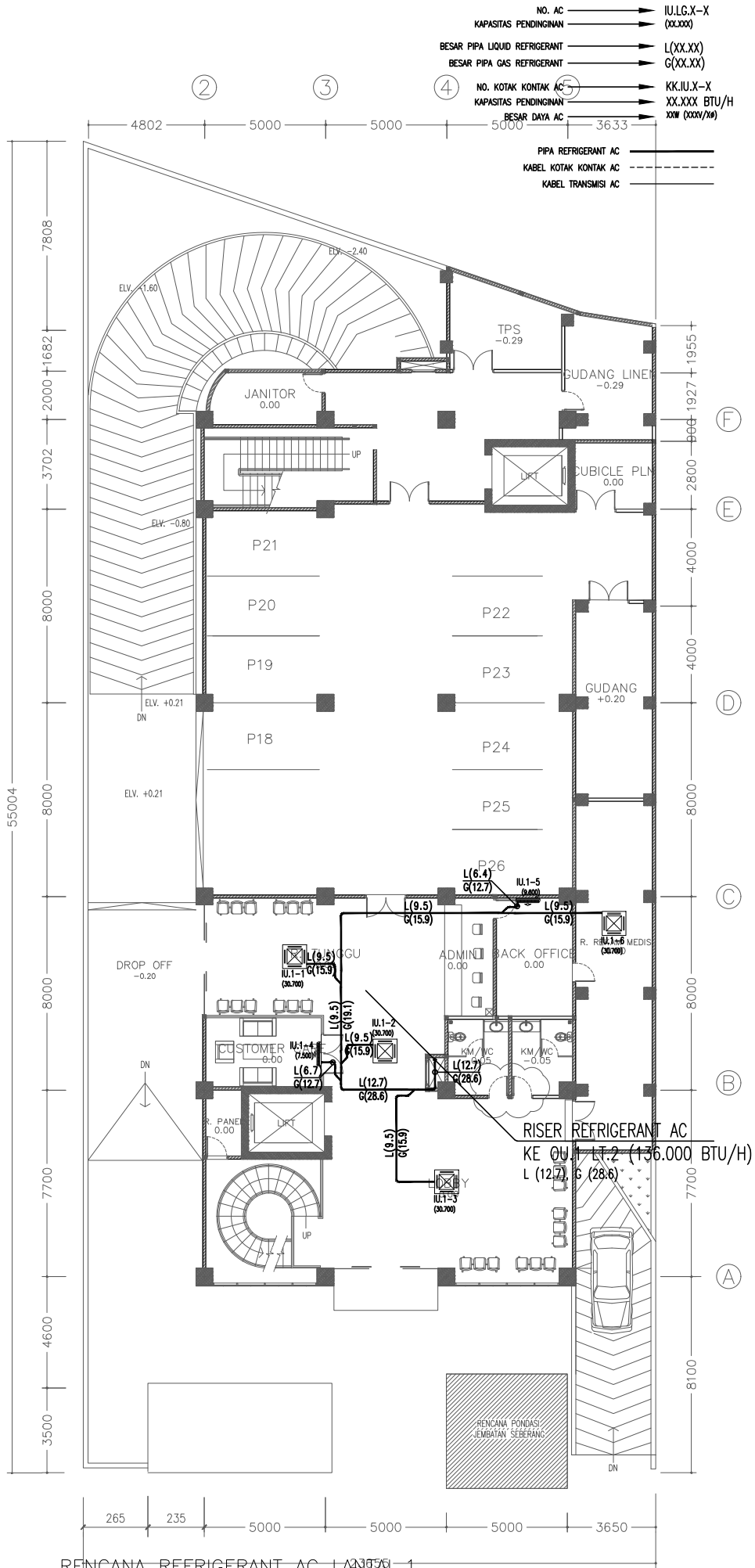
RENCANA REFRIGERANT AC LANTAI 1 SKALA 1:100
