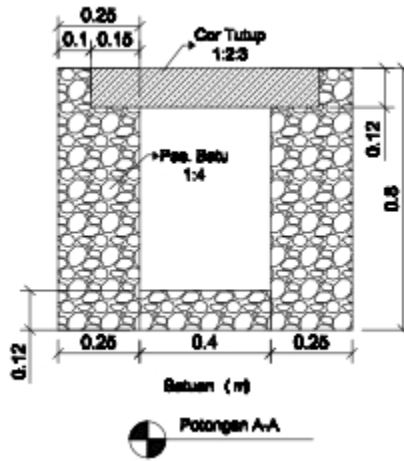
Gambar 2.2. Detail Dainase (Potongan A-A)
