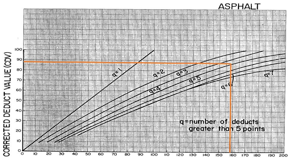
Gambar 12. Grafik CDV STA 6+100 S/D 6+200
