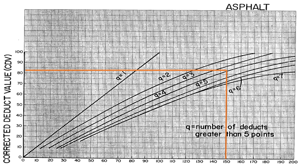
Gambar 10. Grafik CDV STA 5+900 S/D 6+000
