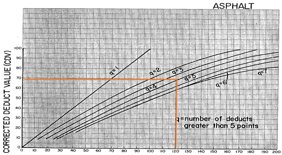
Gambar 37. Grafik CDV STA 8+600 S/D 8+700
