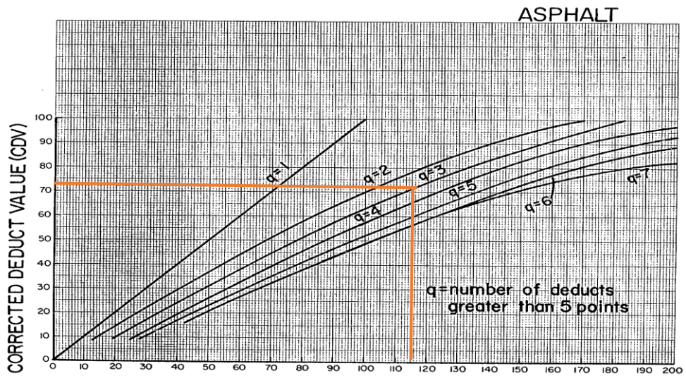
Gambar 7. Grafik CDV STA 5+600 S/D 5+700
