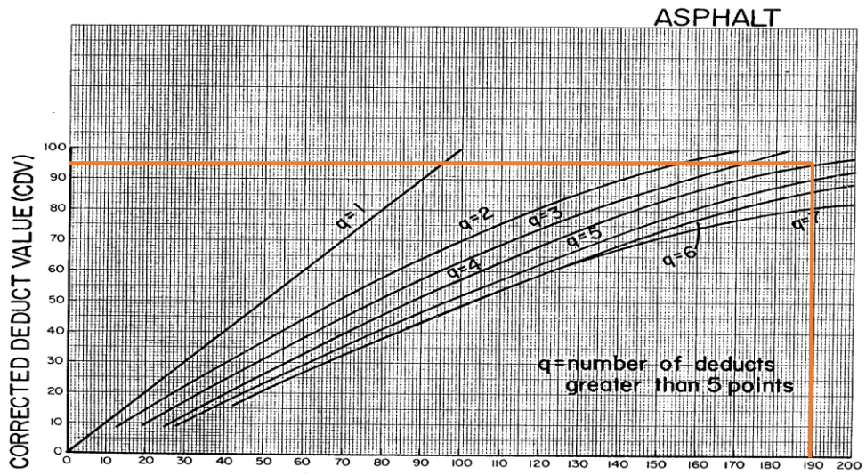
Gambar 24. Grafik CDV STA 7+300 S/D 7+400
