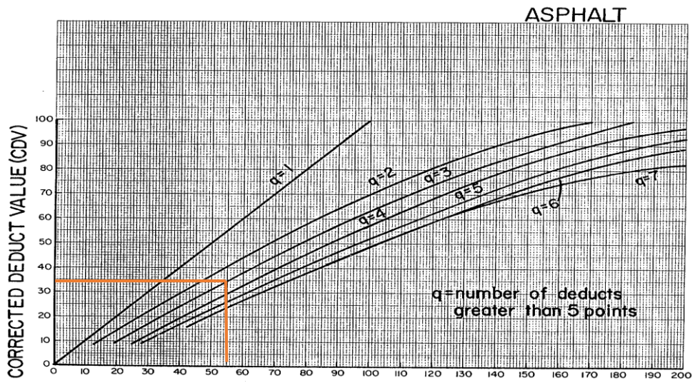
Gambar 23. Grafik CDV STA 7+200 S/D 7+300
