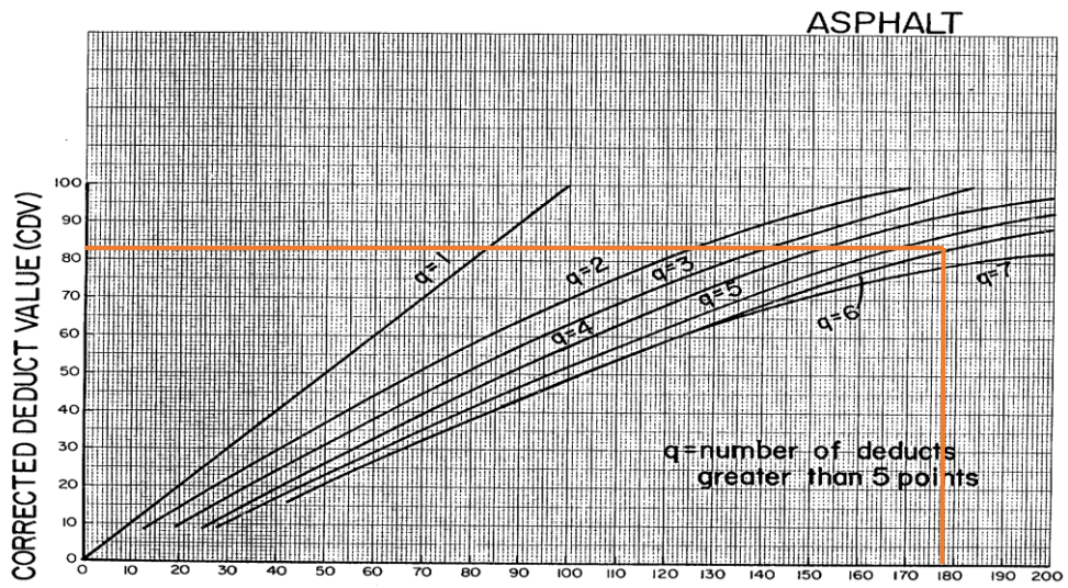
Gambar 13. Grafik CDV STA 6+200 S/D 6+300
