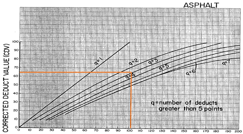
Gambar 11. Grafik CDV STA 6+000 S/D 6+100
