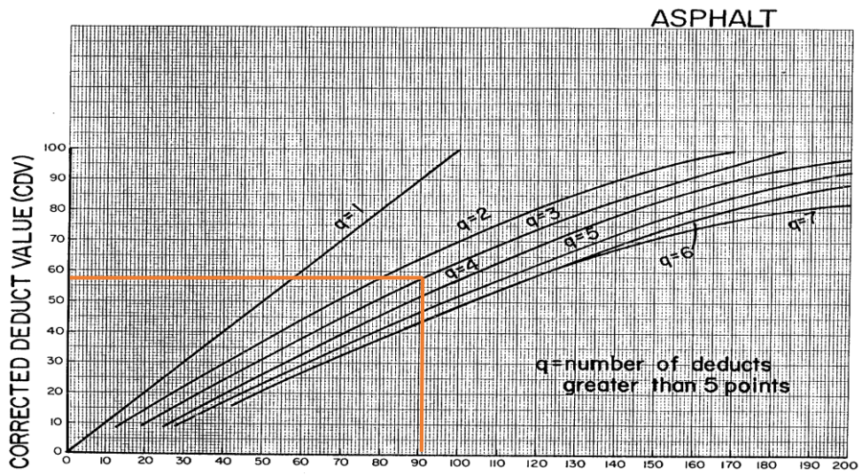
Gambar 21. Grafik CDV STA 7+000 S/D 7+100
