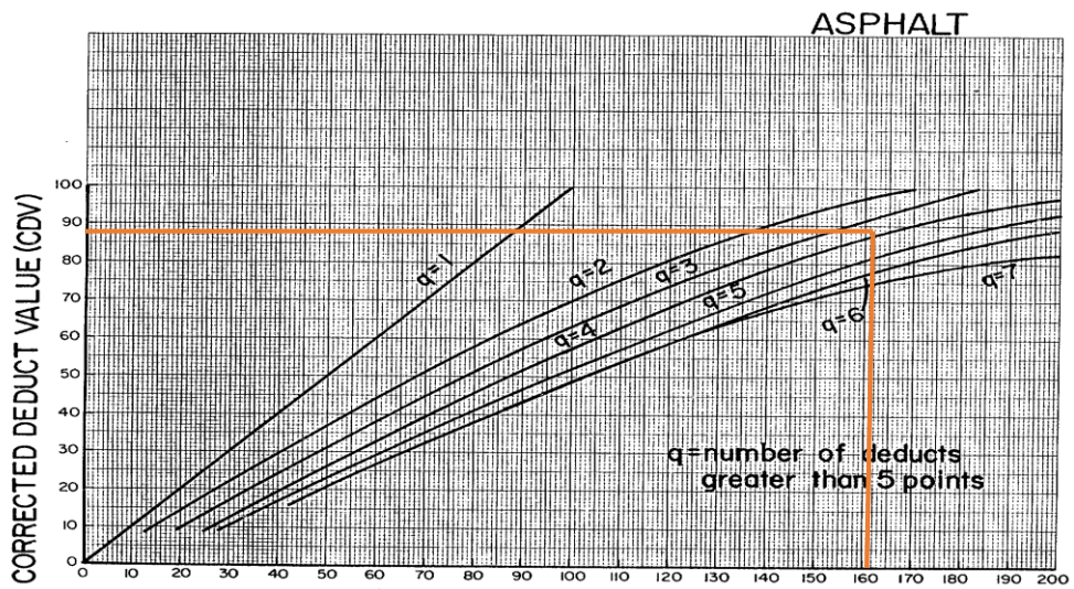
Gambar 14. Grafik CDV STA 6+300 S/D 6+400
