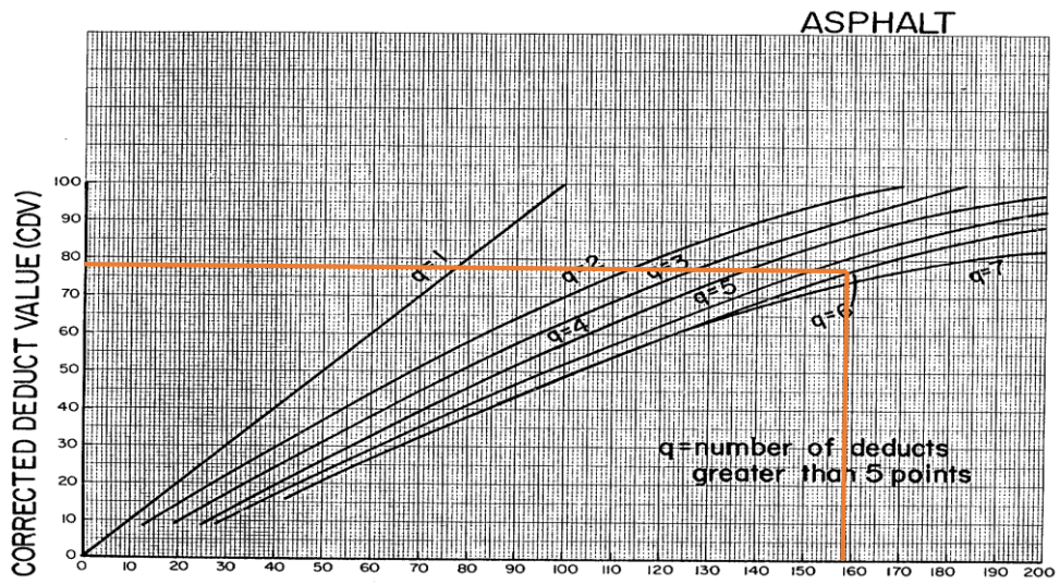
Gambar 35. Grafik CDV STA 8+400 S/D 8+500
