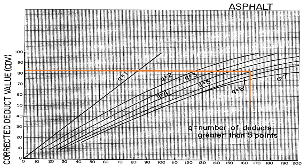
Gambar 30. Grafik CDV STA 7+900 S/D 8+000
