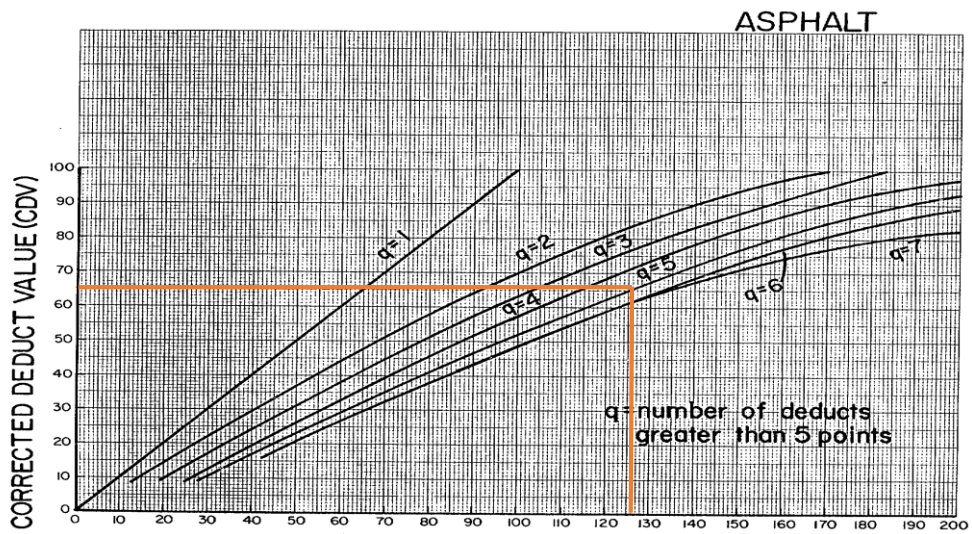
Gambar 28. Grafik CDV STA 7+700 S/D 7+800
