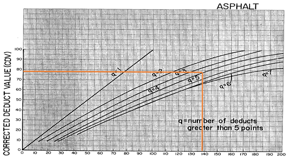
Gambar 22. Grafik CDV STA 7+100 S/D 7+200
