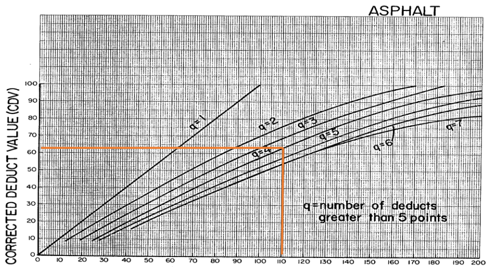
Gambar 40. Grafik CDV STA 8+900 S/D 9+000
