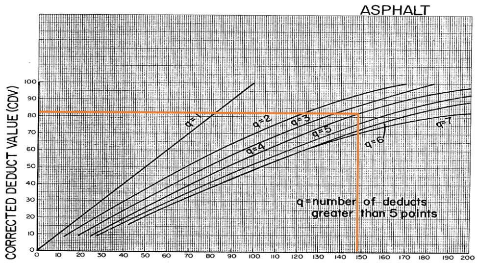
Gambar 25. Grafik CDV STA 7+400 S/D 7+500
