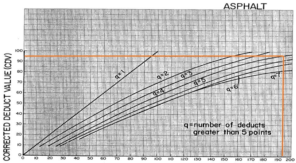
Gambar 41. Grafik CDV STA 9+000 S/D 9+100
