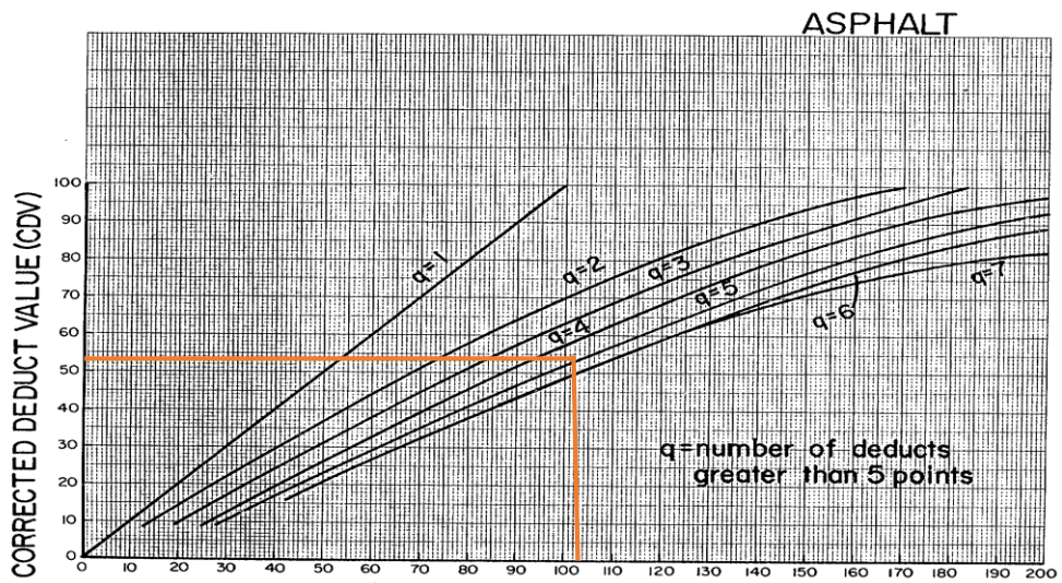
Gambar 36. Grafik CDV STA 8+500 S/D 8+600
