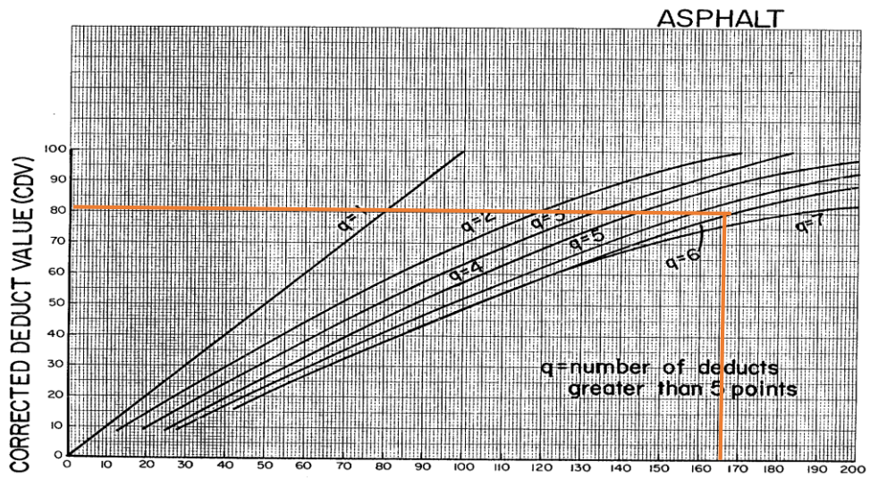
Gambar 39. Grafik CDV STA 8+800 S/D 8+900
