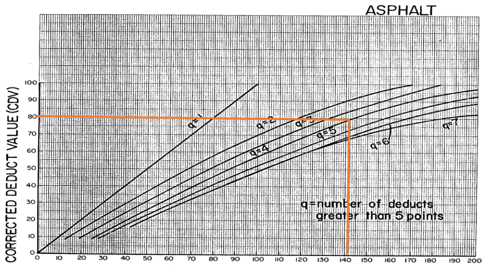
Gambar 5. Grafik CDV STA 5+400 S/D 5+500
