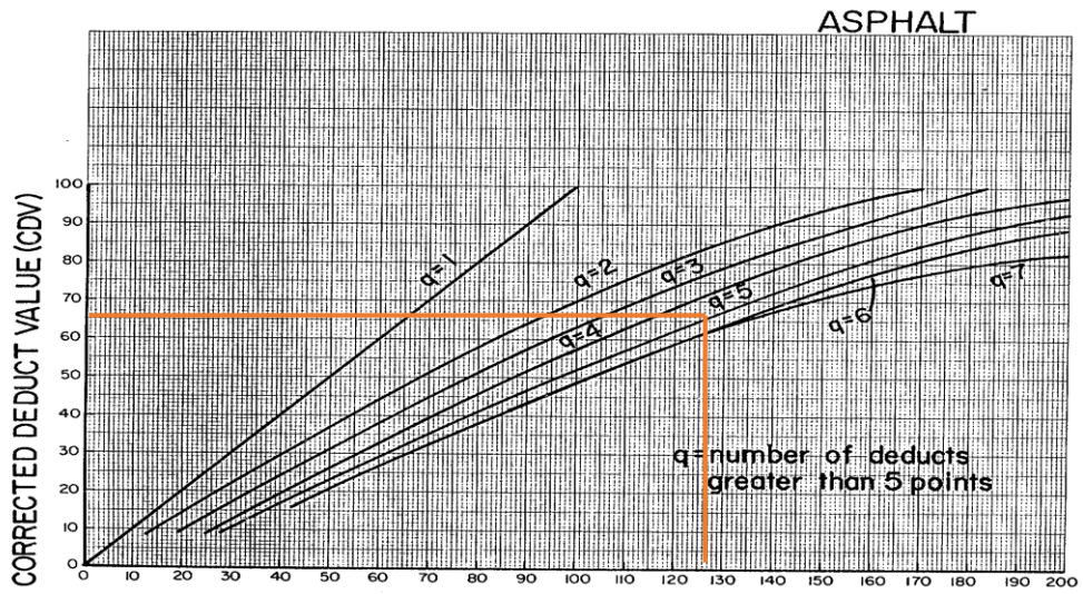
Gambar 42. Grafik CDV STA 9+100 S/D 9+200
