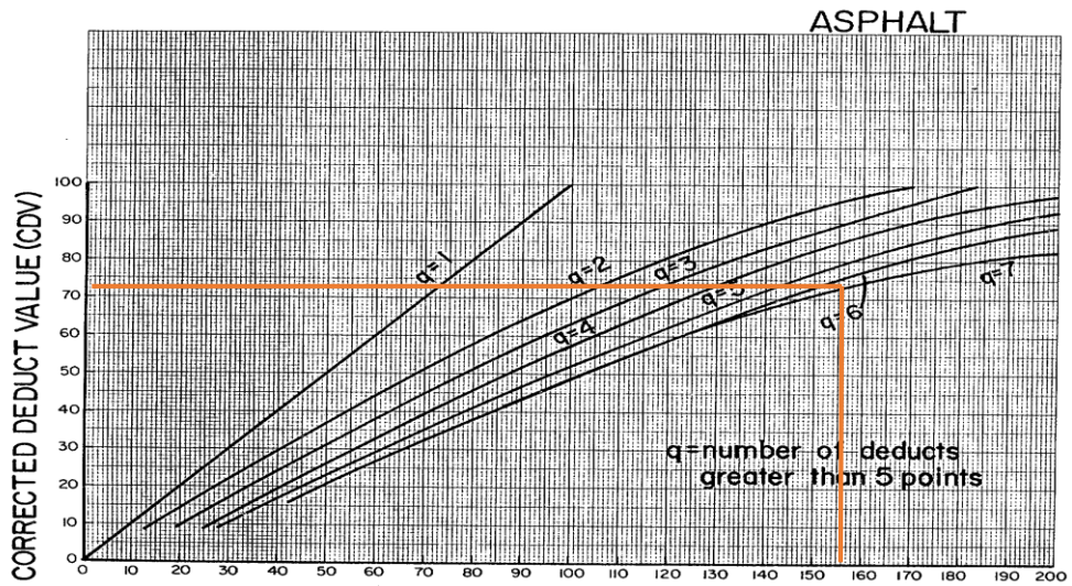
Gambar 6. Grafik CDV STA 5+500 S/D 5+600
