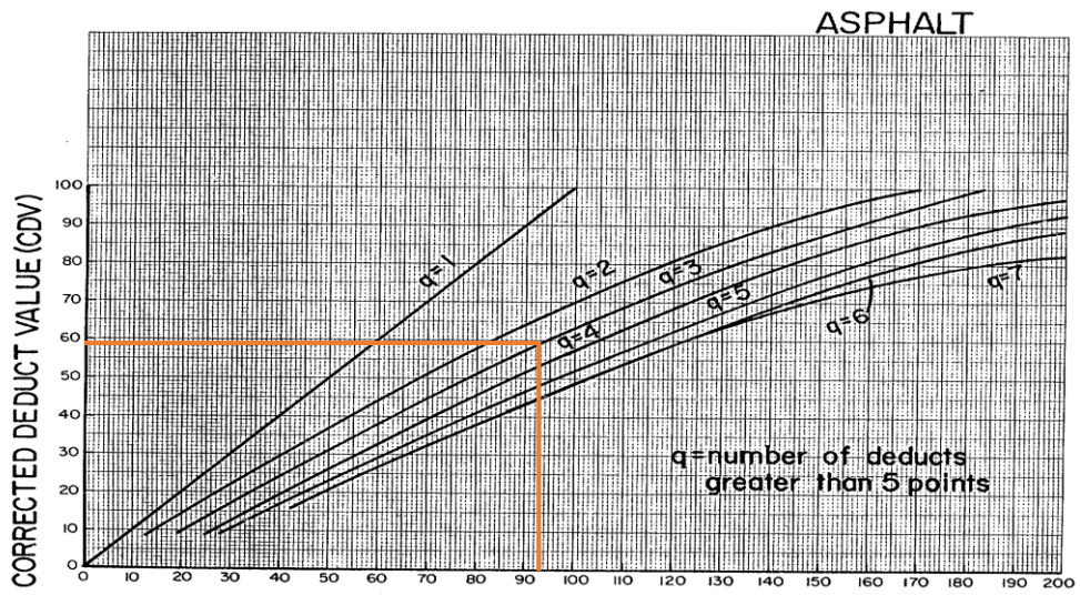
Gambar 33. Grafik CDV STA 8+200 S/D 8+300
