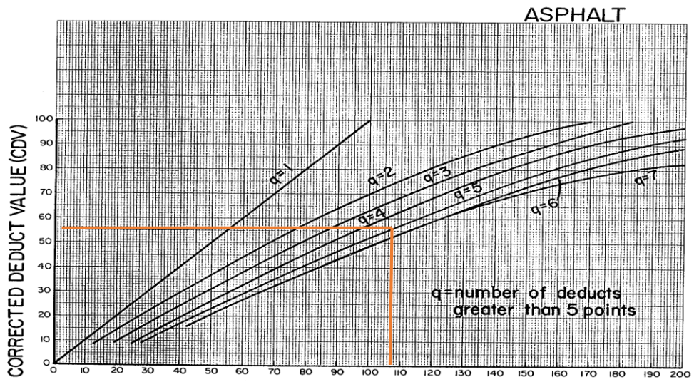
Gambar 31. Grafik CDV STA 8+000 S/D 8+100
