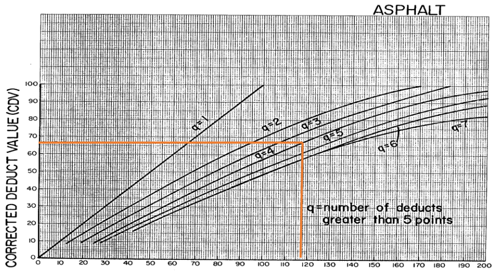
Gambar 34. Grafik CDV STA 8+300 S/D 8+400
