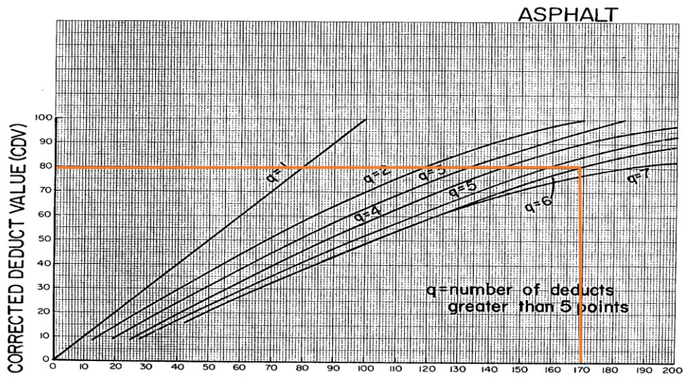
Gambar 15. Grafik CDV STA 6+400 S/D 6+500
