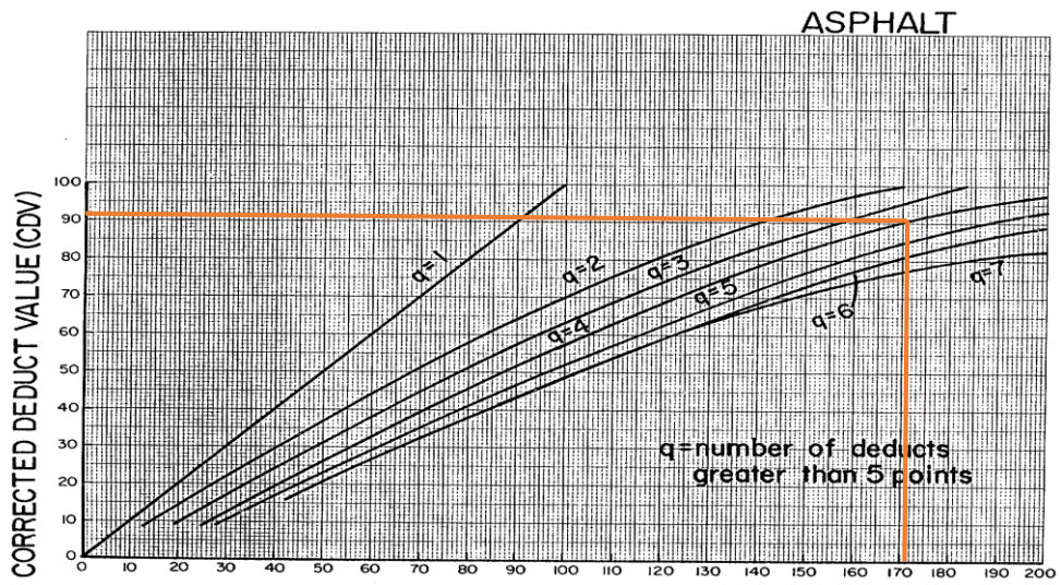
Gambar 27. Grafik CDV STA 7+600 S/D 7+700
