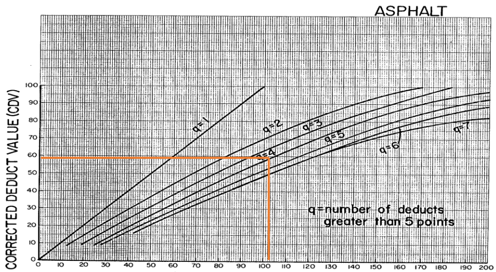
Gambar 16. Grafik CDV STA 6+500 S/D 6+600
