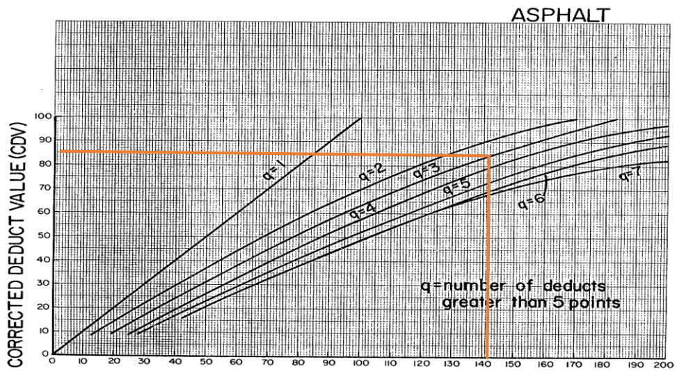
Gambar 26. Grafik CDV STA 7+500 S/D 7+600
