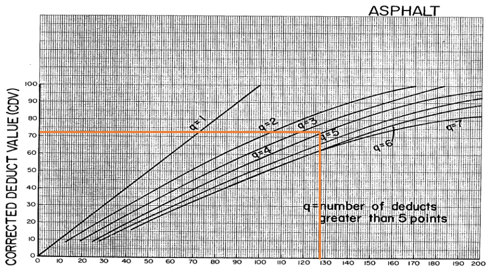
Gambar 18. Grafik CDV STA 6+700 S/D 6+800
