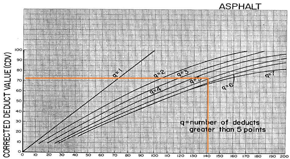
Gambar 44. Grafik CDV STA 9+300 S/D 9+400
