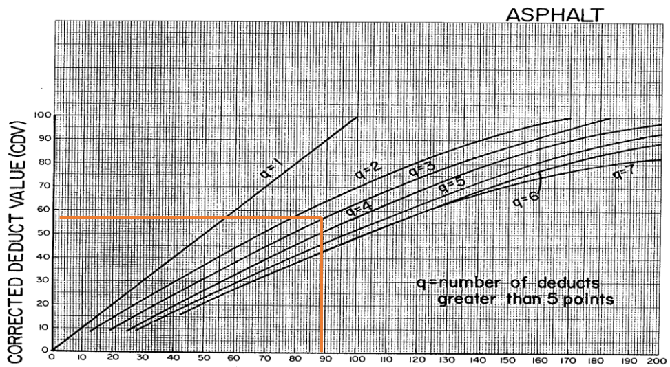
Gambar 32. Grafik CDV STA 8+100 S/D 8+200
