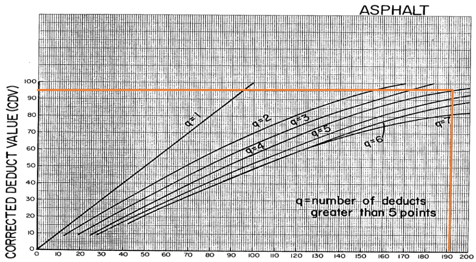
Gambar 43. Grafik CDV STA 9+200 S/D 9+300
