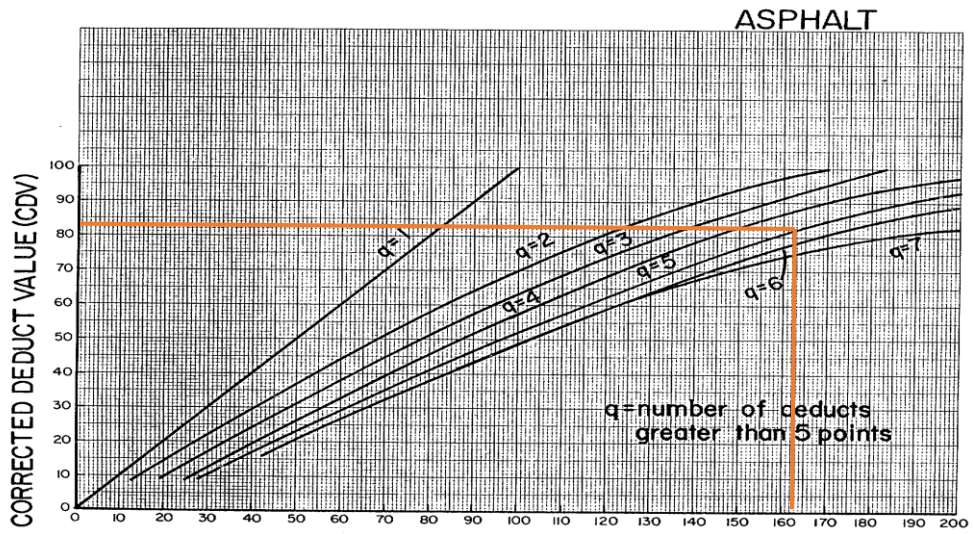
Gambar 38. Grafik CDV STA 8+700 S/D 8+800
