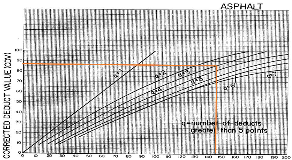
Gambar 20. Grafik CDV STA 6+900 S/D 7+000
