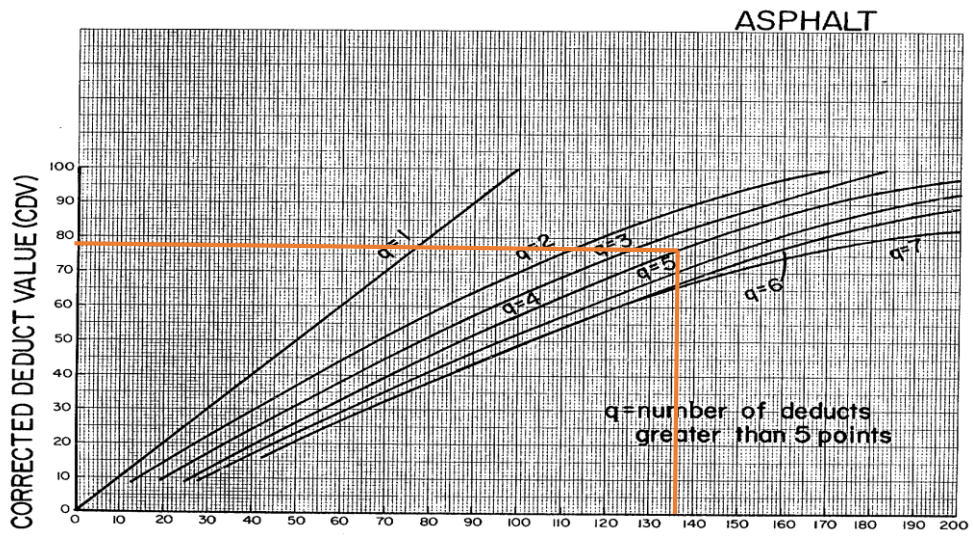
Gambar 19. Grafik CDV STA 6+800 S/D 6+900
