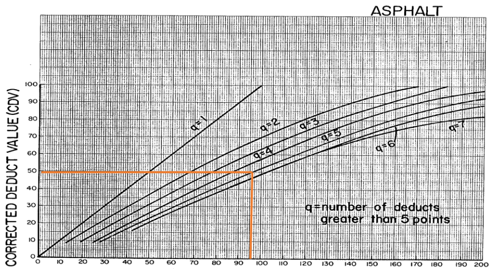
Gambar 4. Grafik CDV STA 5+300 S/D 5+400
