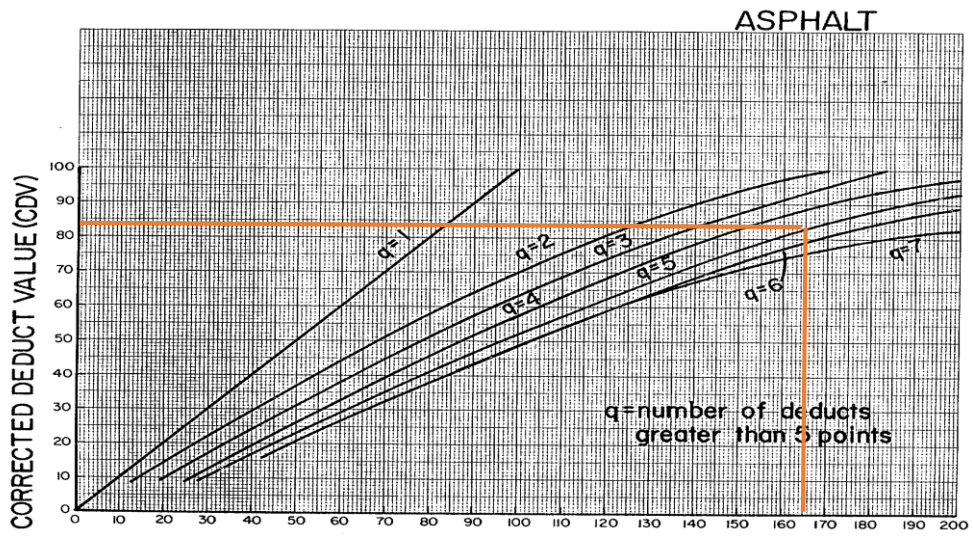
Gambar 29. Grafik CDV STA 7+800 S/D 7+900
