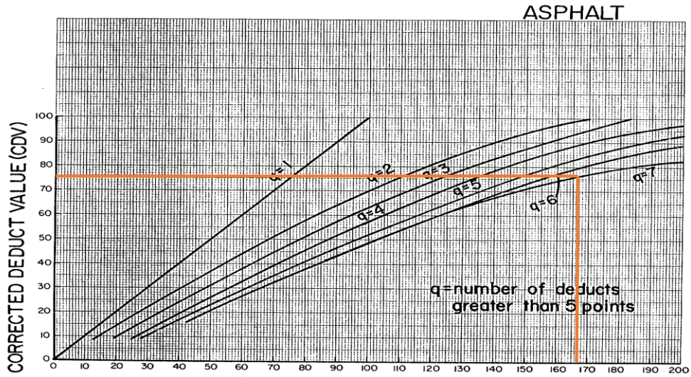
Gambar 1. Grafik CDV STA 5+000 S/D 5+100
