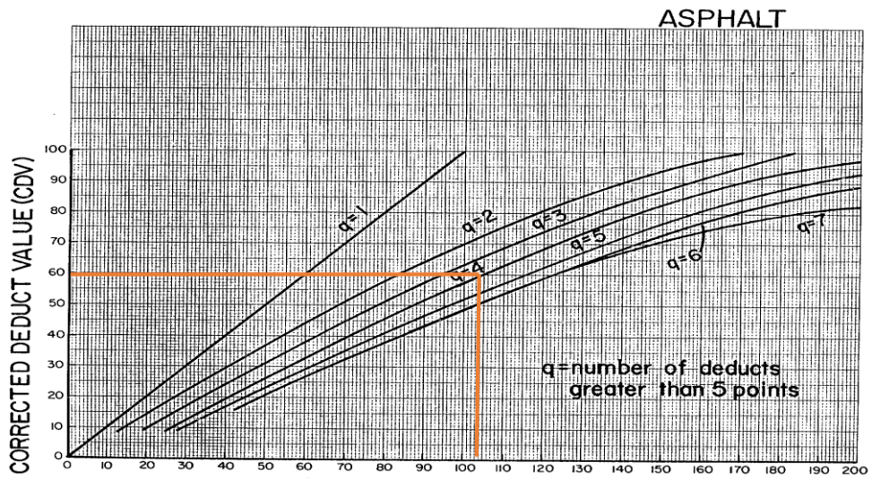
Gambar 17. Grafik CDV STA 6+600 S/D 6+700
