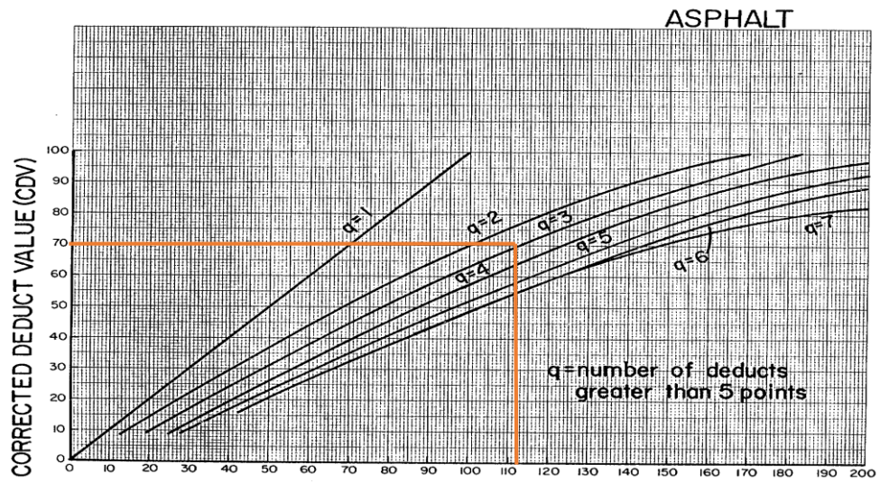
Gambar 45. Grafik CDV STA 9+400 S/D 9+500
