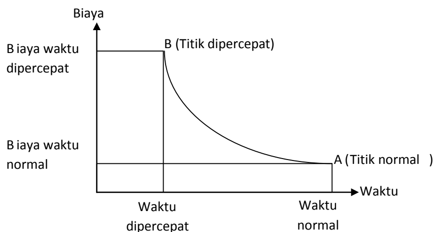
Grafik 3.2 Grafik Hubungan waktu dengan biaya normal dan dipercepat untuk suatu kegiatan (Sumber: Soeharto, 1997).
