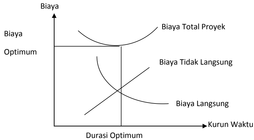
Grafik 3.3 Grafik Hubungan waktu dengan biaya total, biaya langsung, dan biaya tak langsung (Sumber: Soeharto, 1997)
