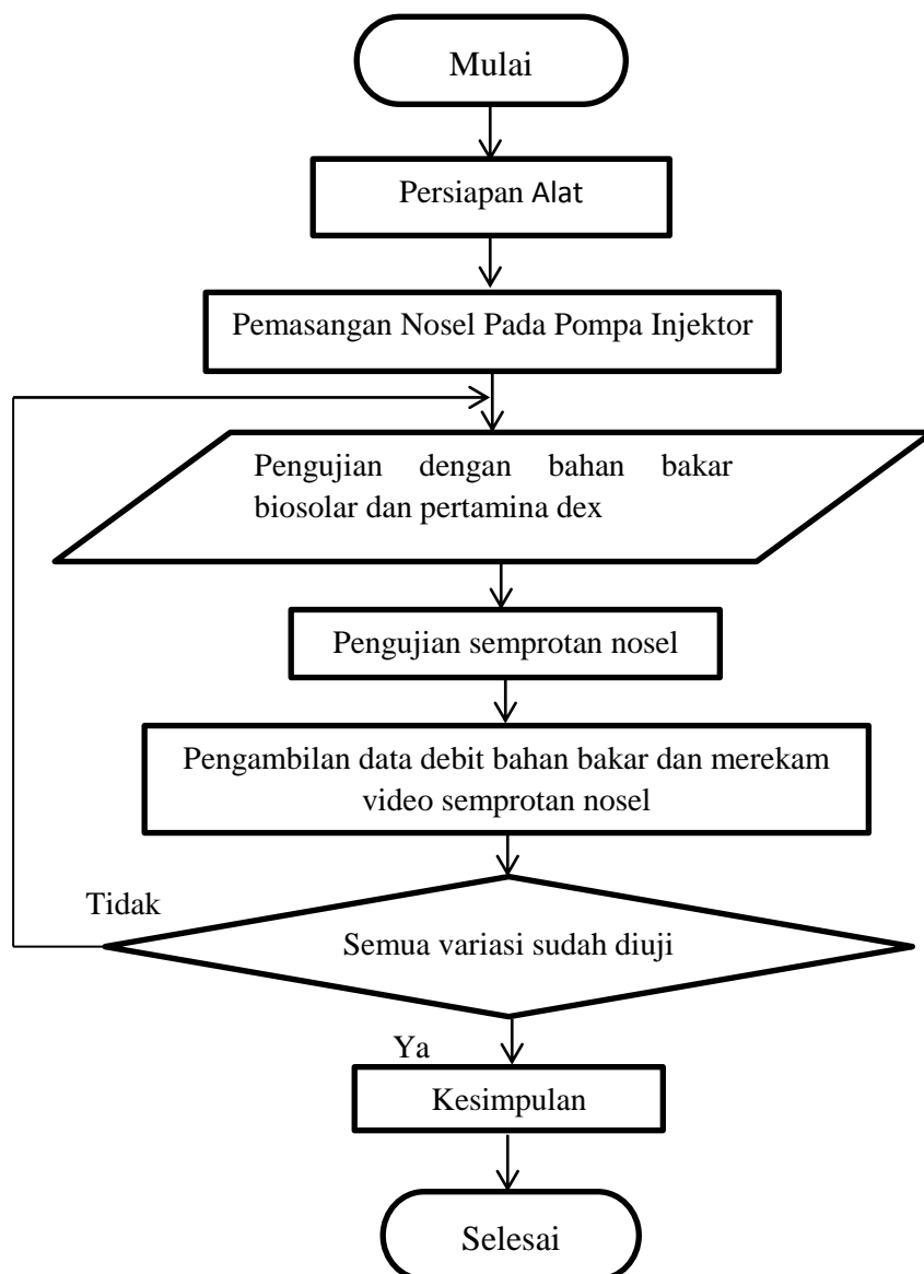
Gambar 3.15 Diagram alir pengujian karakteristik injeksi
