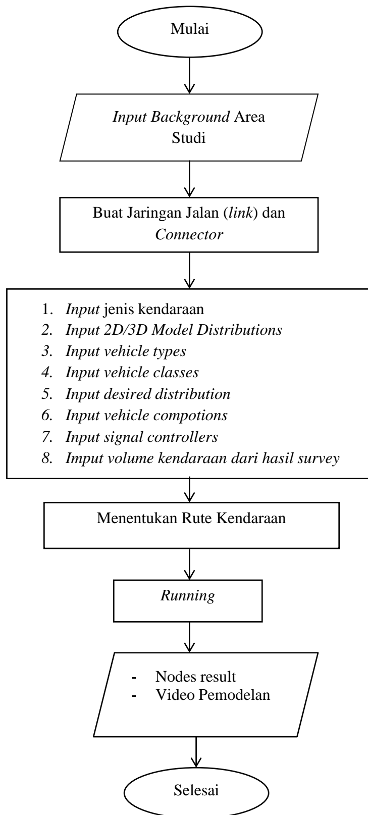
Gambar 4.4 Diagram Alir Proses Analisis Data dengan VISSIM 9.00-03
