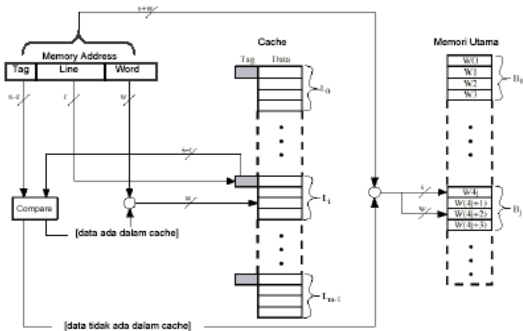
Gambar 7.7 Pemetaan Langsung
