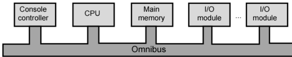
Gambar 2. 4 Struktur Bus DEC - PDP-8
