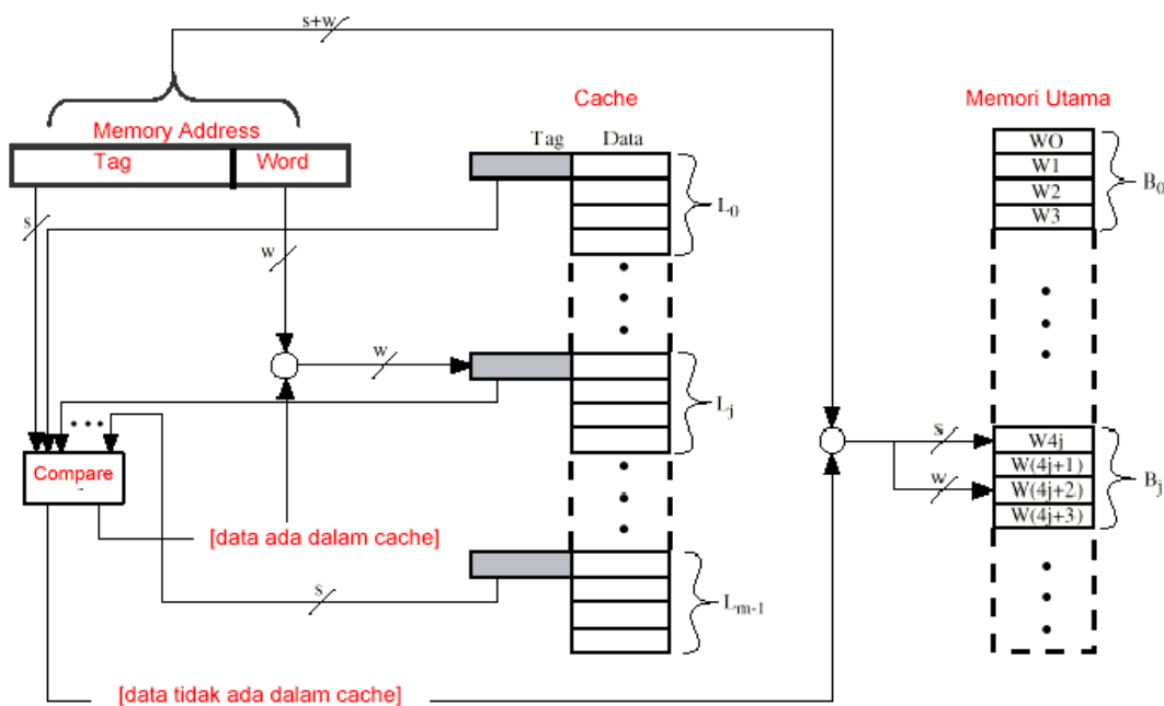
Gambar 7.8 Pemetaan Asosiatif
