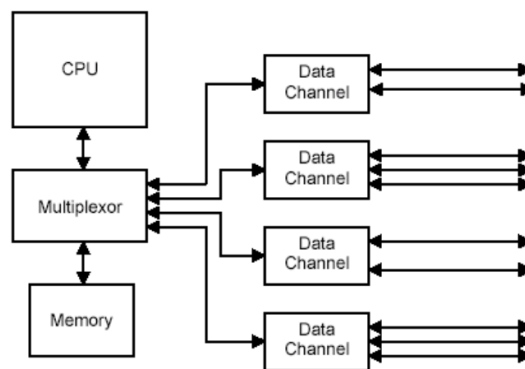
Gambar 2.3 Konfigurasi IBM 7094
