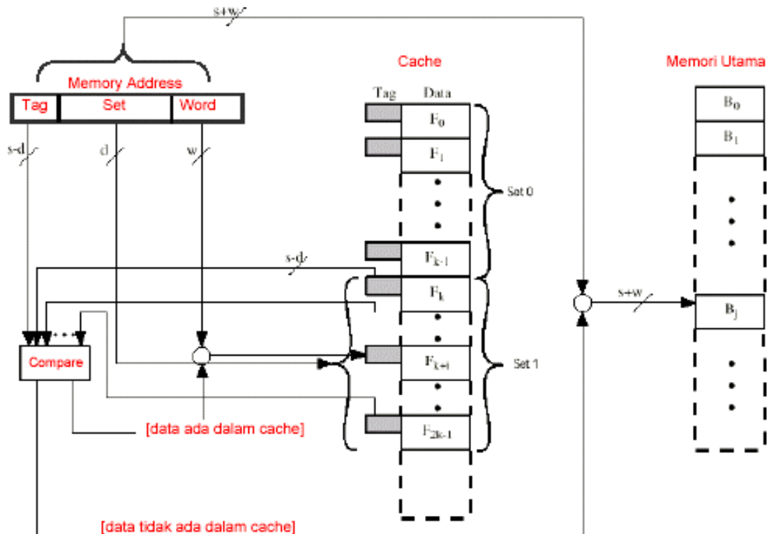
Gambar 7.9. Pemetaan Asosiatif Set
