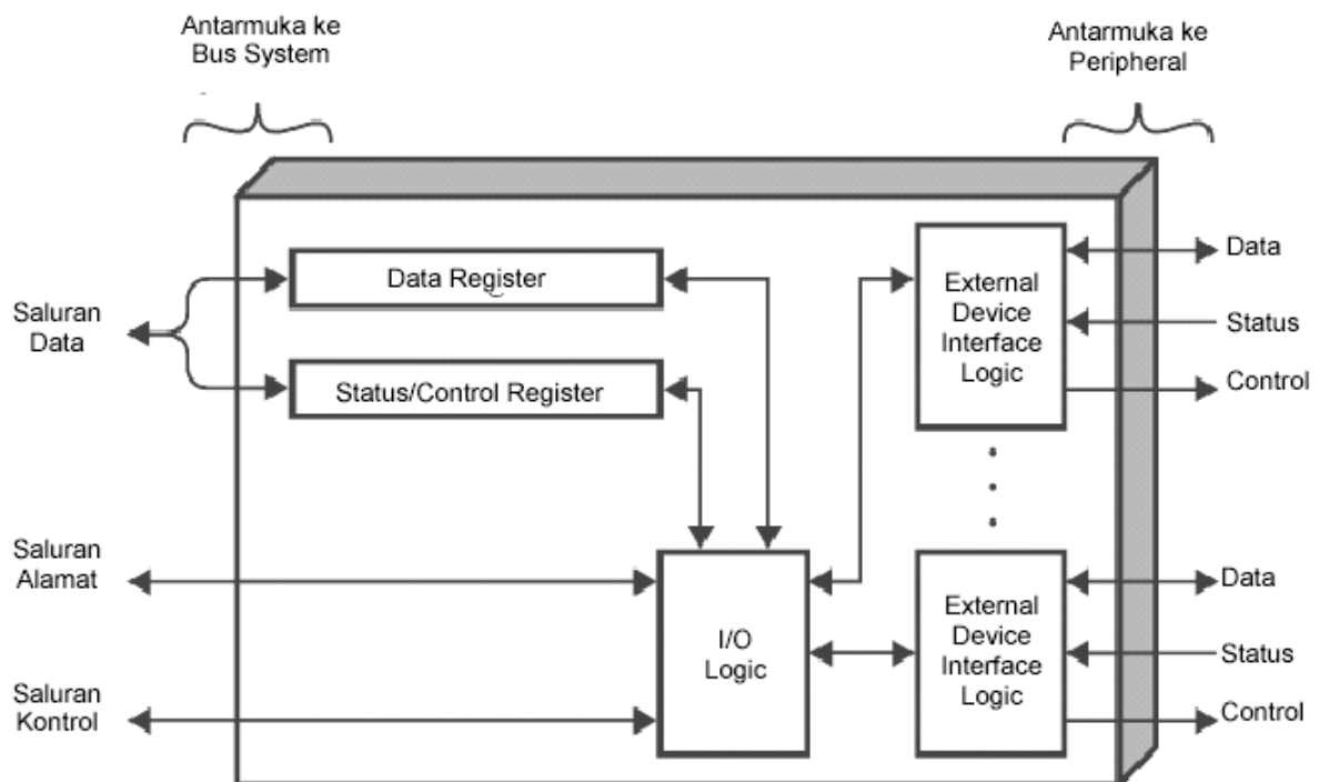
Gambar 8.2. Blok diagram struktur modul I/O
