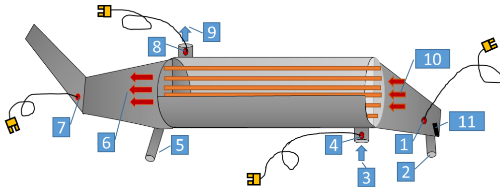
Gambar 3.15 Skema kondensor
