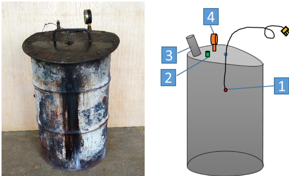
Gambar 3.16 reaktor
