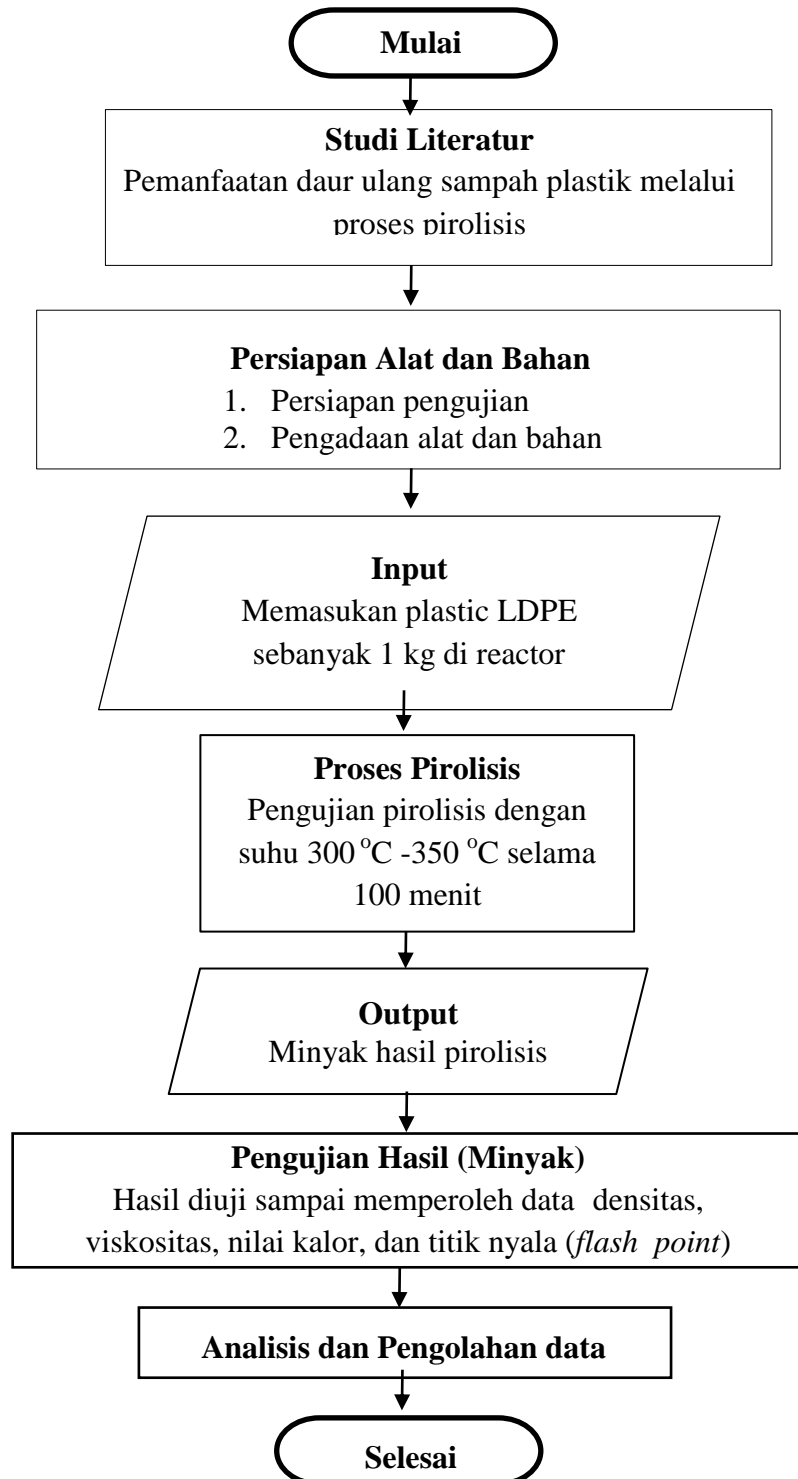
Gambar 3.21. Diagram alir pengujian
