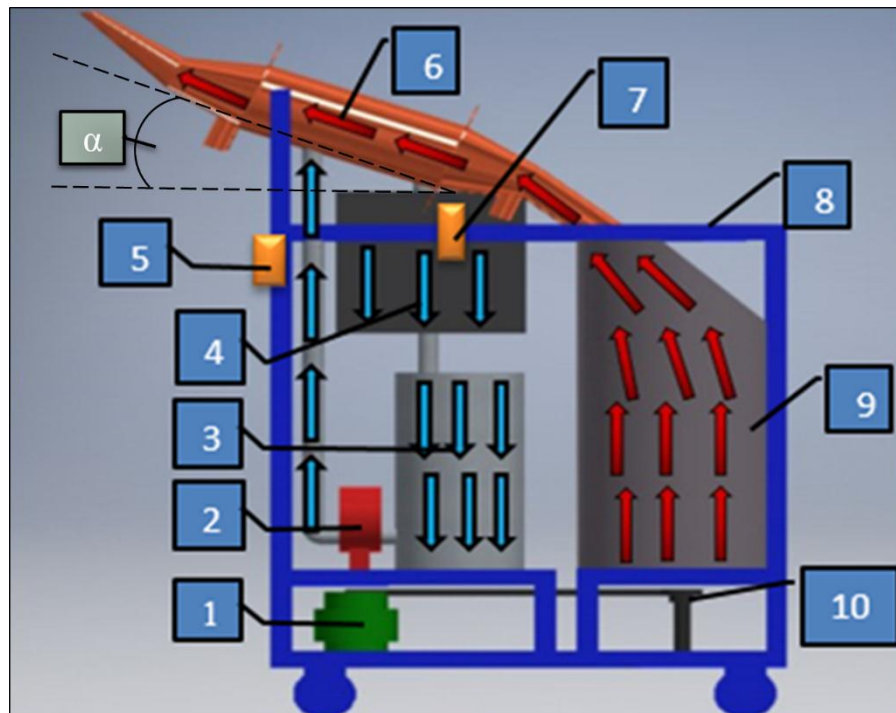
Gambar 3.3 Skema alat Pirolisis
