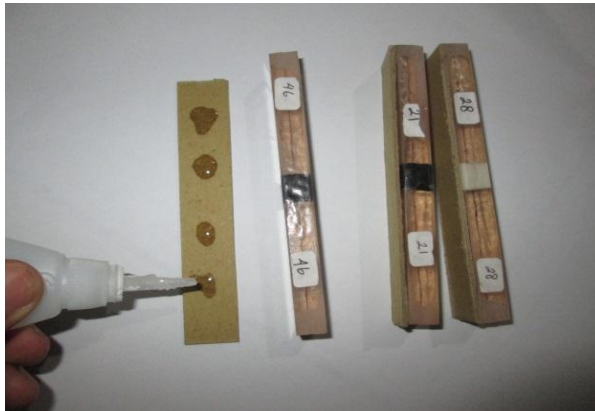
Gambar 3.28 Pengeleman spesimen dengan karton
