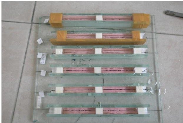
Gambar 3.25 Penuangan resin
