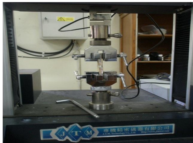
Gambar 3.13 Alat uji tarik
