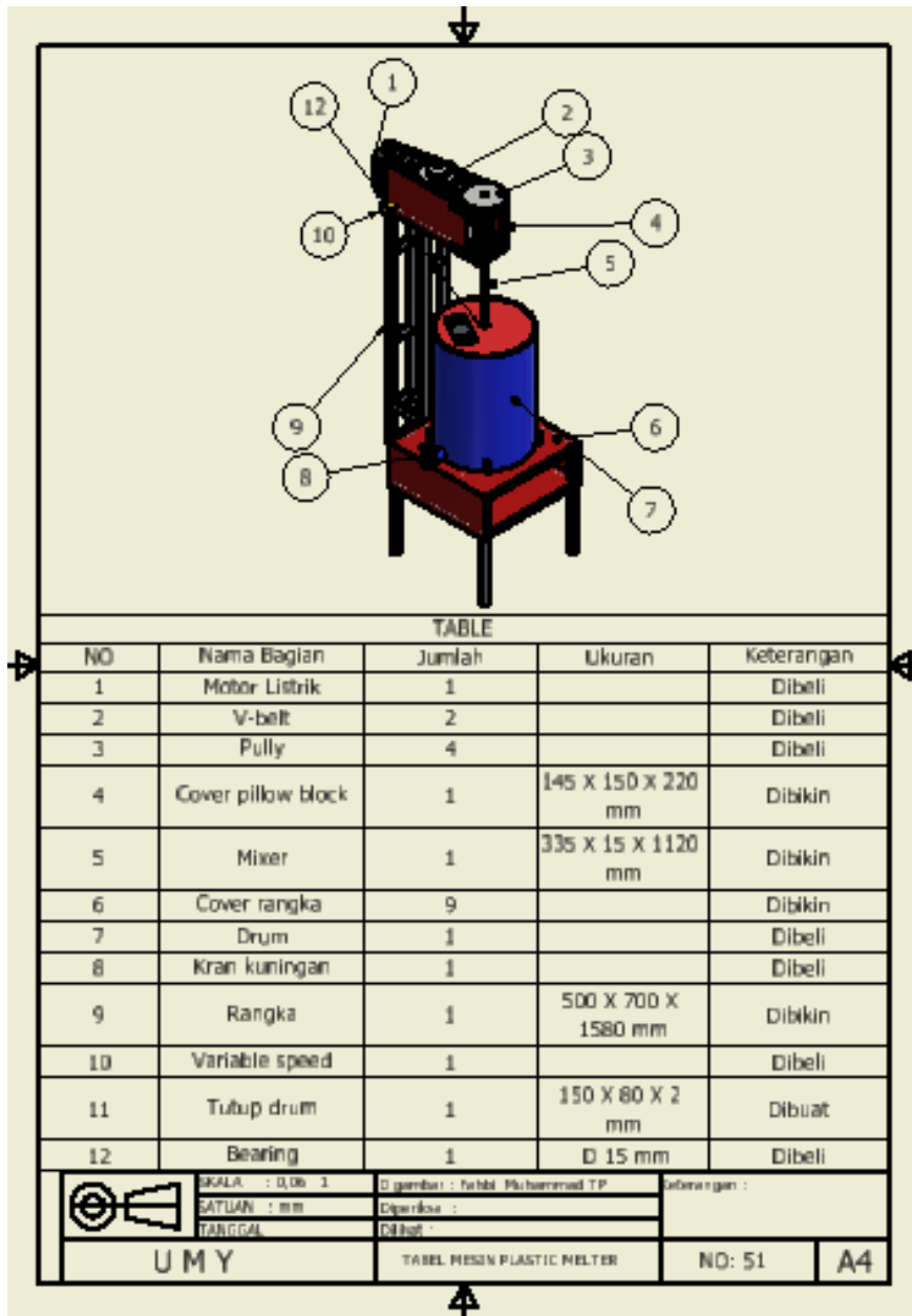
Gambar komponen-komponen mesin plastic melter
