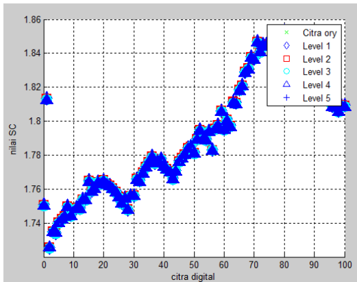
Gbr. 12 Parameter SC untuk Pyramida Gaussian
