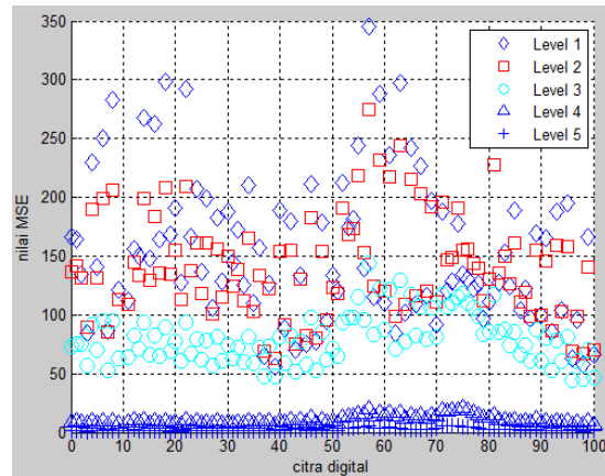
Gbr. 10 Parameter MSE untuk Pyramida Gaussian
