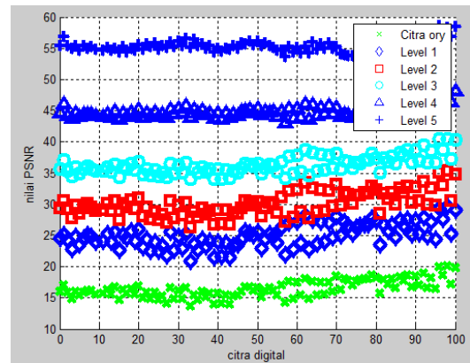
Gbr. 14 Parameter PSNR untuk Pyramida Gaussian
