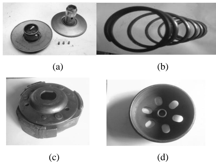
Gambar 2.11 Komponen Puli Sekunder (Rochadi, 2009)
