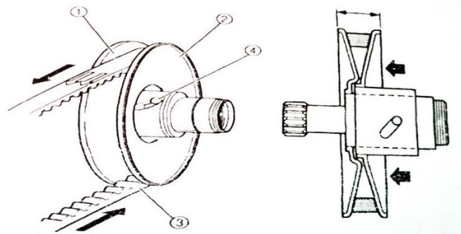
Gambar 2.14 Torsi cam pada saat mendaki dan akselerasi (Pujiyanto, 2014)
