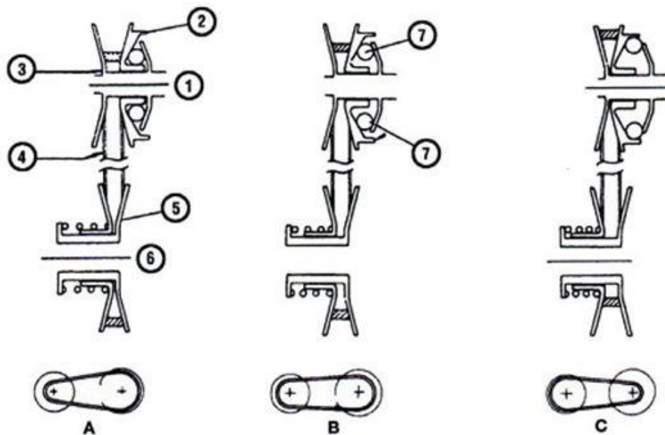
Gambar 2.12 Posisi dan Cara Kerja Puli (Rochadi, 2009)
