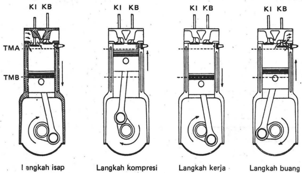
Gambar 2.1 Skema Gerakan Torak 4 Langkah (Arismunandar, 2002)
