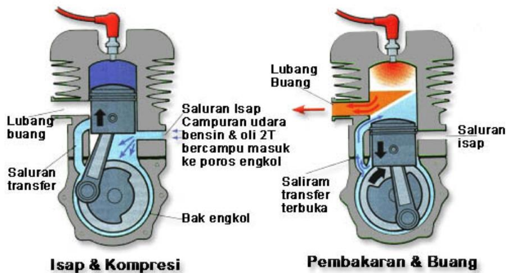
Gambar 2.6 Skema Gerakan Torak 2 Langkah (Jama, 2008)
