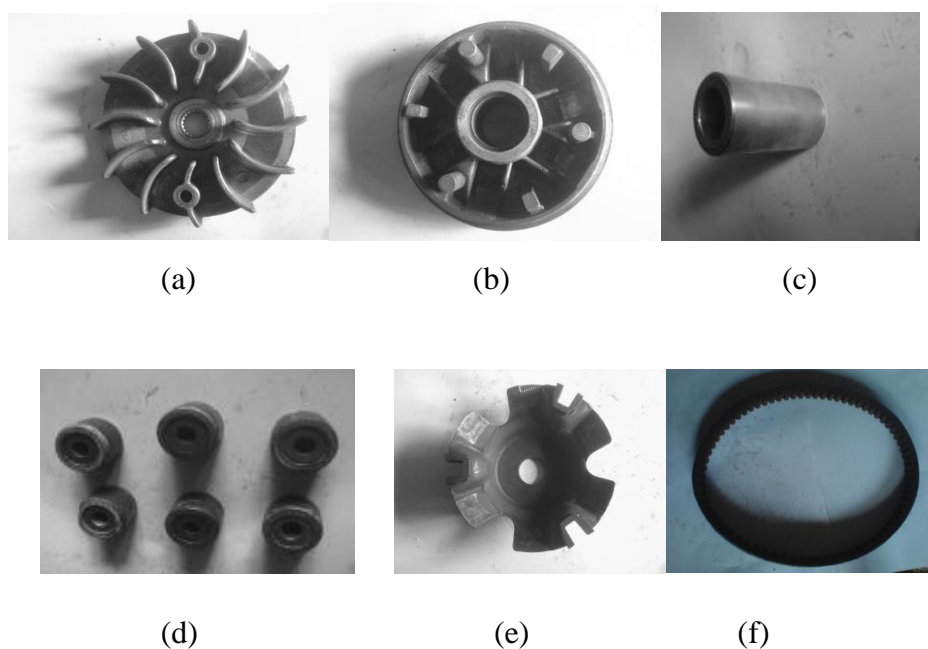
Gambar 2.10 Komponen Puli Primer (Rochadi, 2009)
