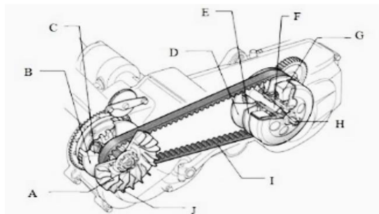
Gambar 2.9 Transmisi Otomatis (Pujiyanto, 2014)
