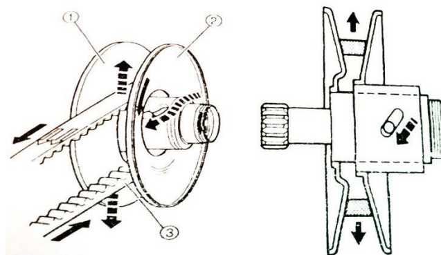
Gambar 2.13 Torsi cam pada beban ringan (Pujiyanto, 2014)
