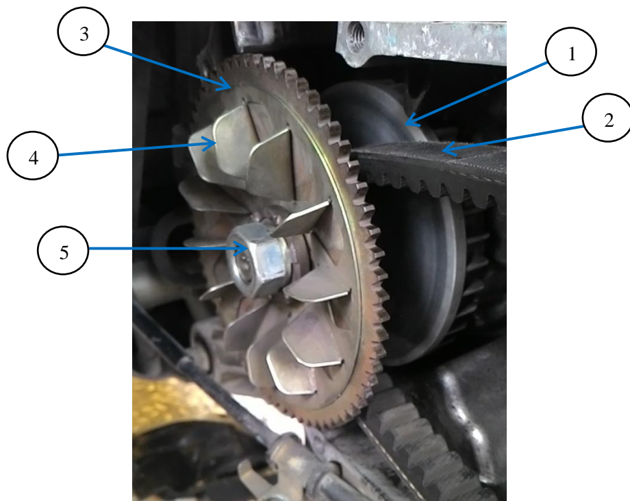
Gambar 3.7 Konstruksi Pada Puli Primer
