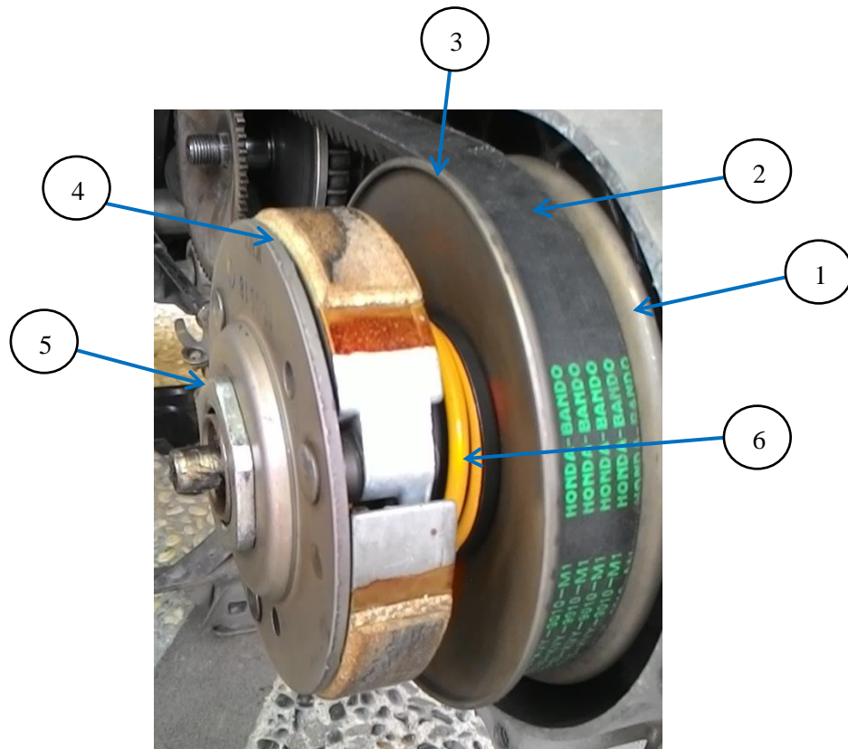
Gambar 3.8 Konstruksi Pada Puli Sekunder
