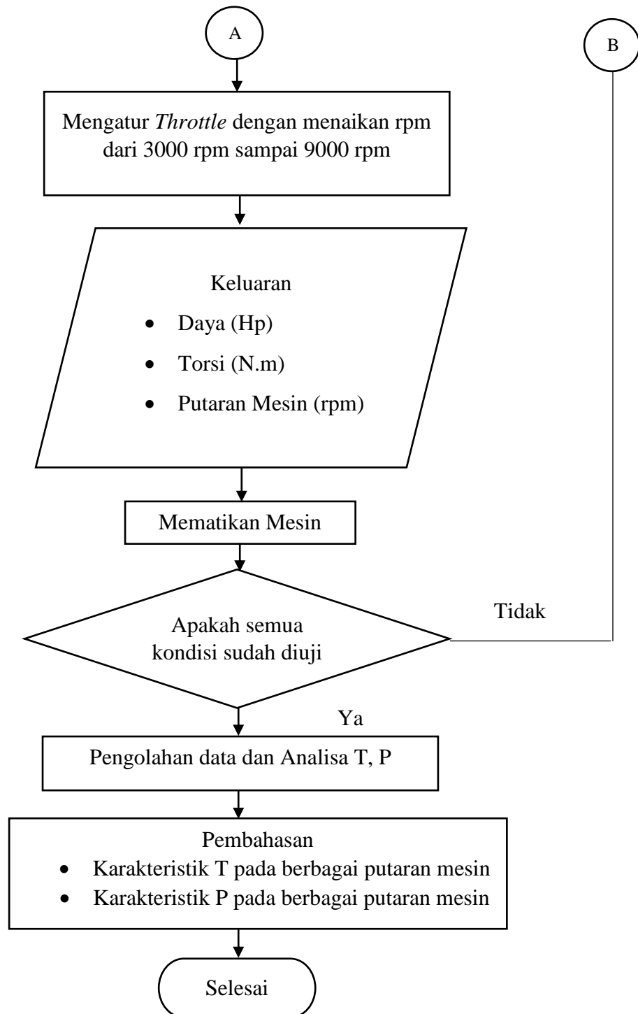
Gambar 3.9 Flow Chart Pengujian Daya dan Torsi (Lanjutan)
