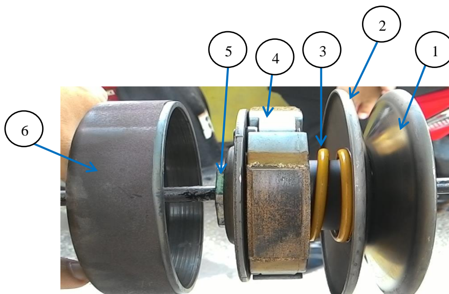
Gambar 3.4 Komponen Pada Puli Sekunder
