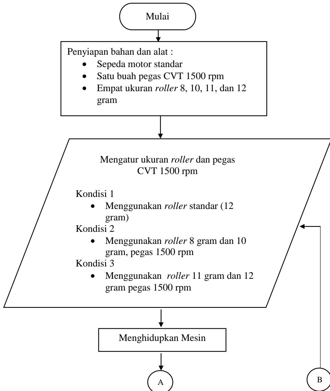
Gambar 3.9 Flow Chart Pengujian Daya dan Torsi
