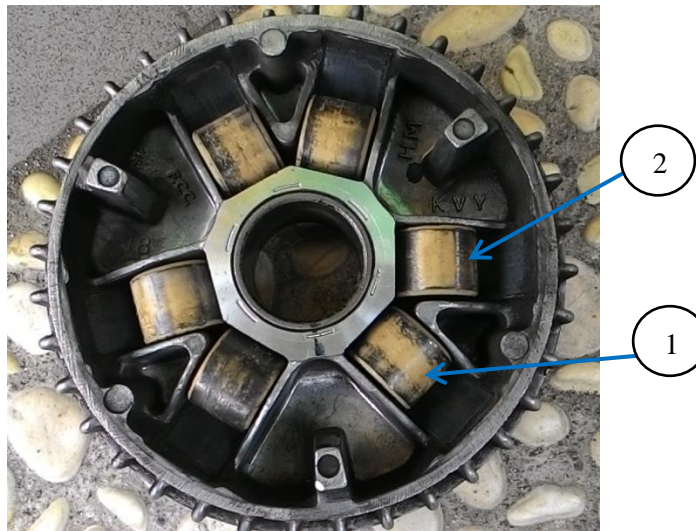
Gambar 3.5 Pemasangan Kombinasi Roller
