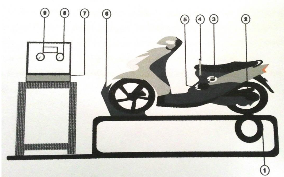
Gambar 3.10 Skema Alat Uji Daya dan Torsi Motor
